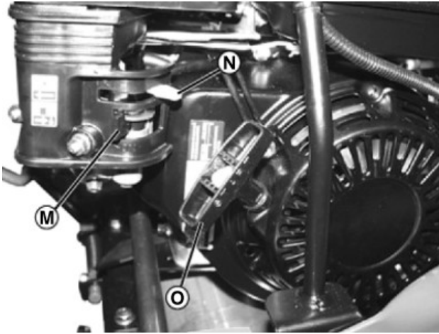
Commandes moteur
