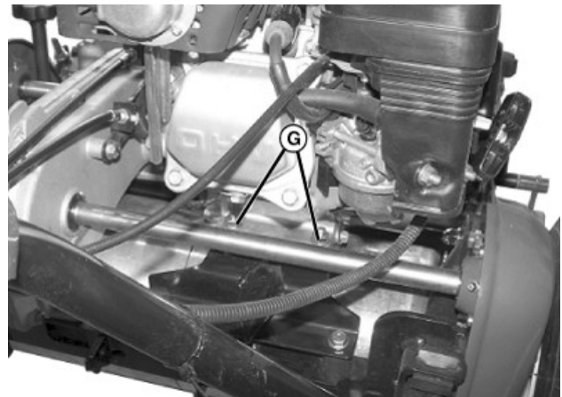
엔진의 후면
