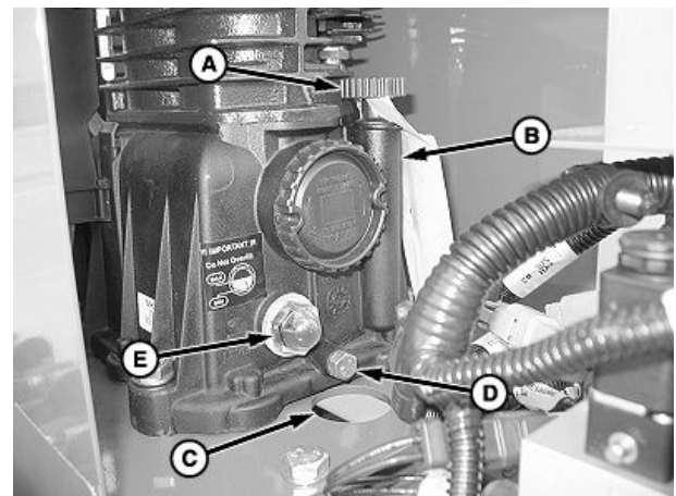
A—Cobertura B—Reservatório C—Orifício de Drenagem
