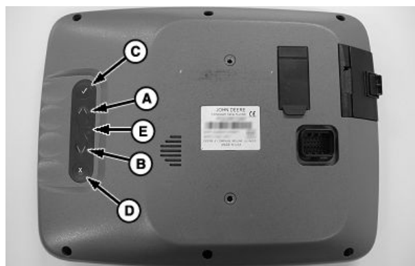
Controles Manuais do GreenStar™ 2100 e do GreenStar™ 2600
