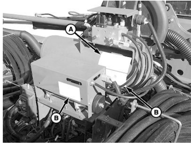
Tanque de Ar da Força Descendente Pneumática - Plantadeiras Integrais (Força Descendente com um Único Ponto de Ajuste)
