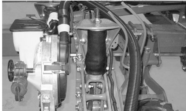
Mola a Ar Devidamente Enrolada (Linha Dupla)
