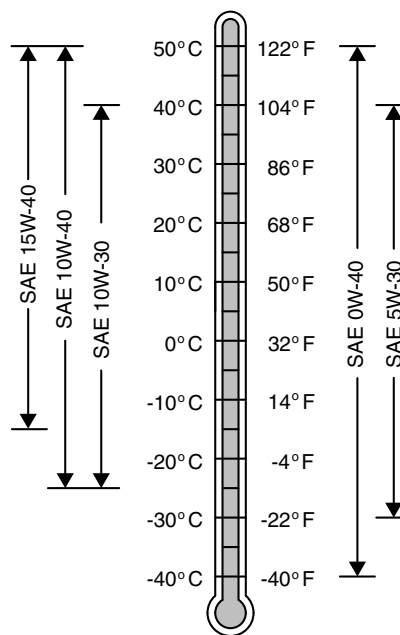
Viscosités d'huile pour différentes températures extérieures
