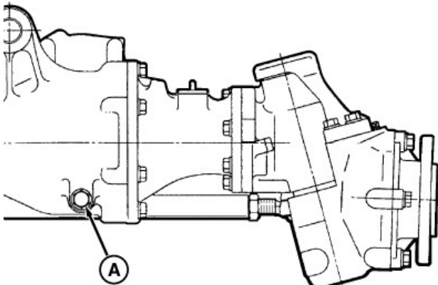
Pohled zezadu na nápravu (pravá strana)
