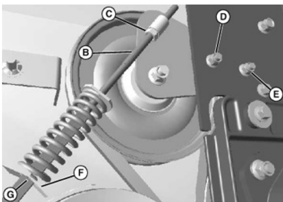
TCAL44930—UN—28MAR13 (Frontmähwerk dargestellt, Seitenmähwerk ähnlich)
