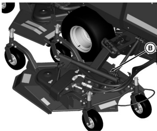
B—Unità di taglio e tiranterie
