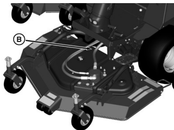
B—Unità di taglio e tiranterie
