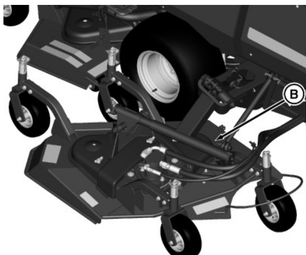
B—Unités de coupe et tringleries
