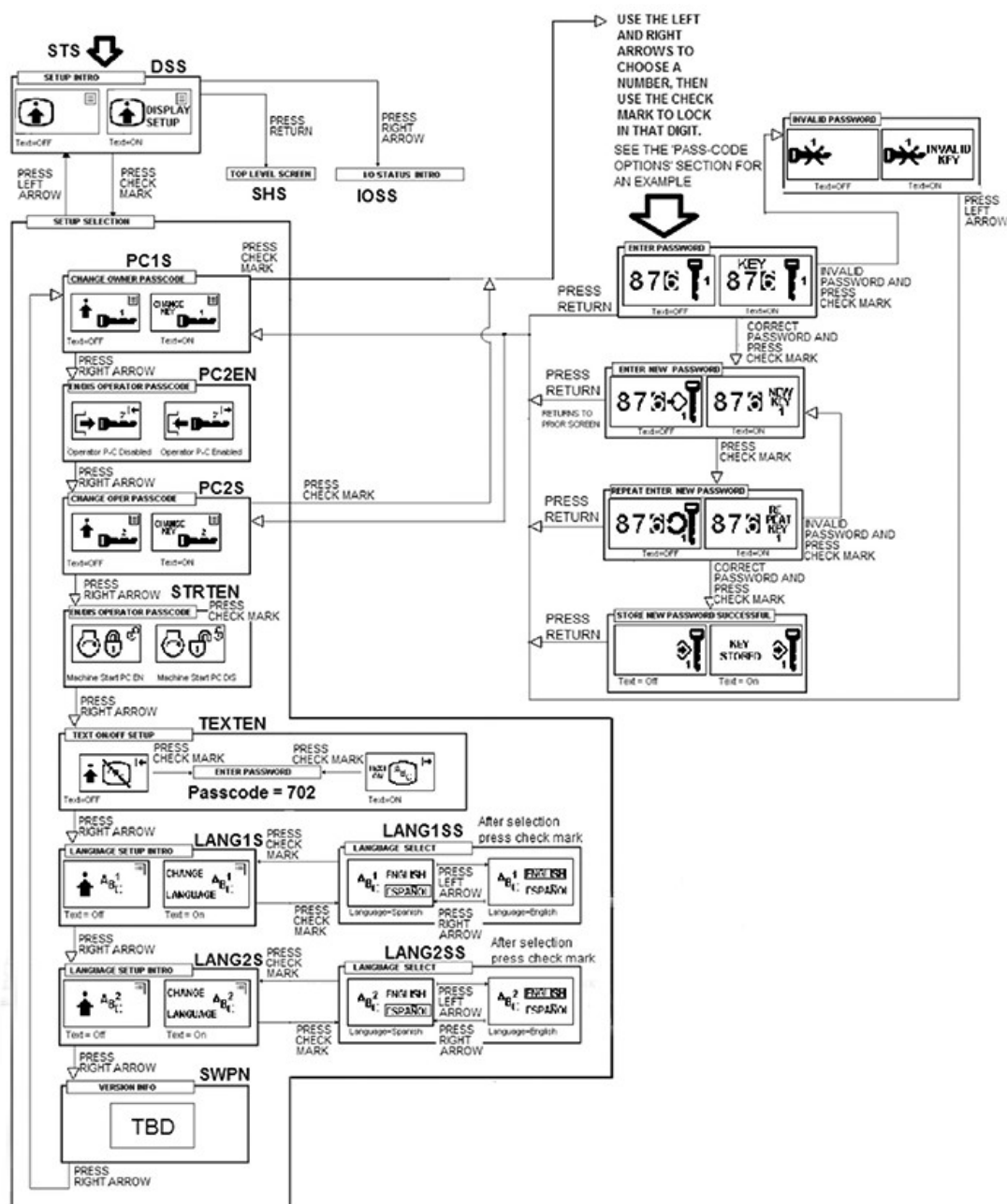
显示器设置流程图
