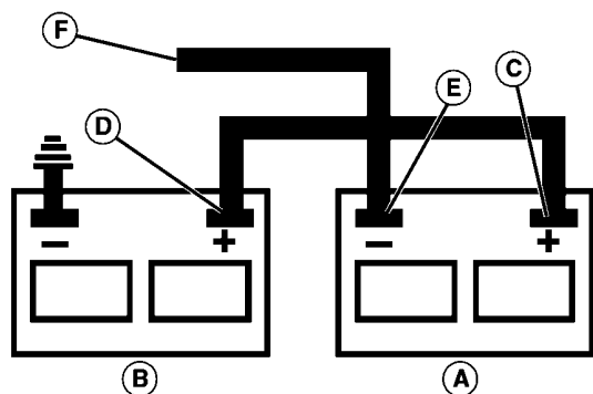
A—Akumulator pomocniczy
