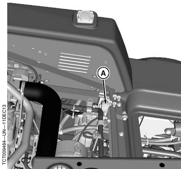
משאבת ההגבר החשמלית נמצאת מתחת למושב בצד שמאל של המכונה.
