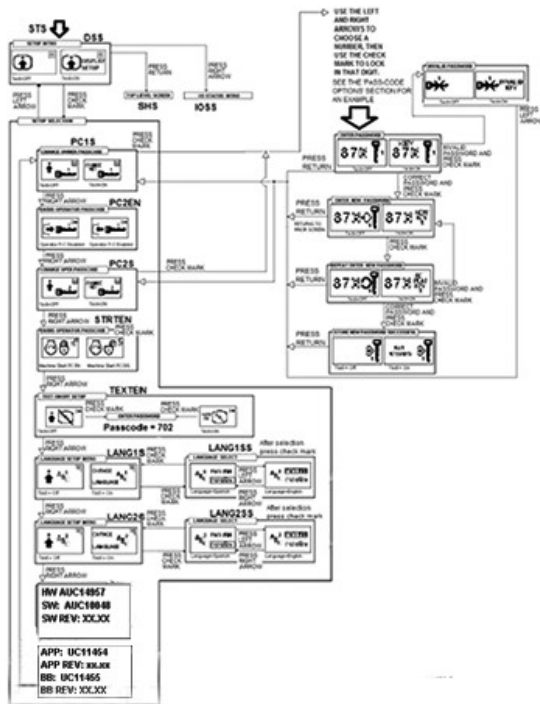
APY42011—UN—25AUG20 Vývojový diagram nastavení displeje
