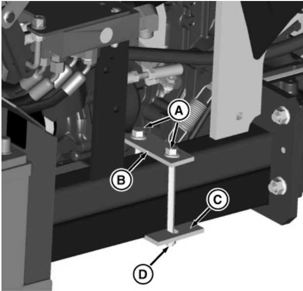
A—Vis M10 X 130 B—Plaque C—Plaque de fixation D—Écrou de blocage, M10
