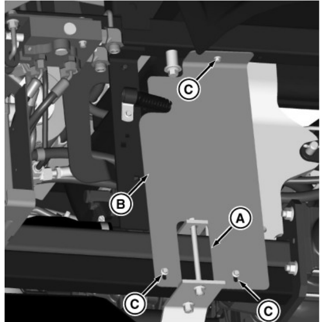
A—Fente de la tôle de protection B—Garant droit C—Vis autotaraudeuses
