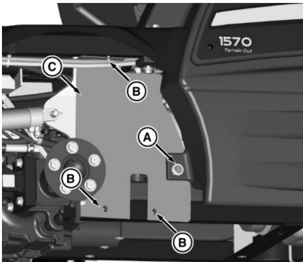
A—Boulonnerie du réservoir de carburant B—Vis autotaraudeuses C—Garant latéral gauche
