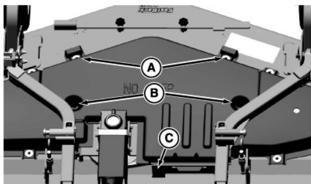
TC102123—UN—27JUN22 Note de l'illustration: Unité de coupe 72 in à décharge arrière illustrée
