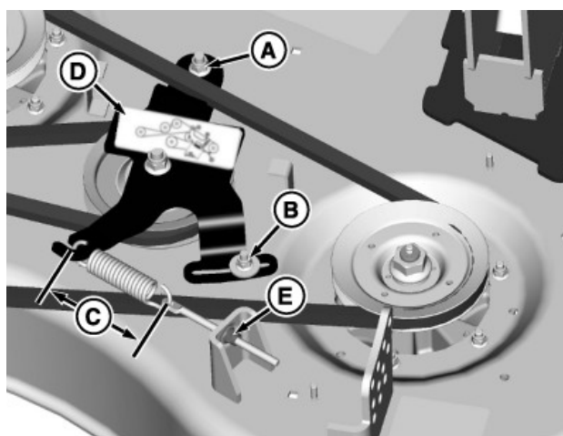
TCT008966—UN—27FEB14 Unité de coupe à décharge latérale de 60 po illustrée, les autres sont similaires.
