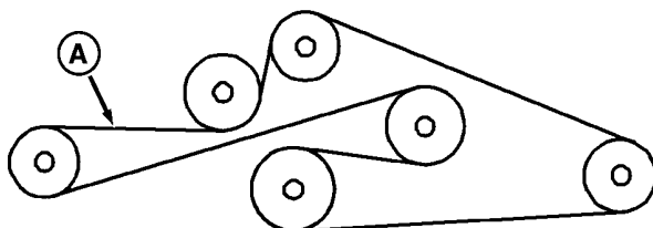
TCT008976—UN—07OCT13 Note de l'illustration: Vue de l'arrière de l'unité de coupe.
