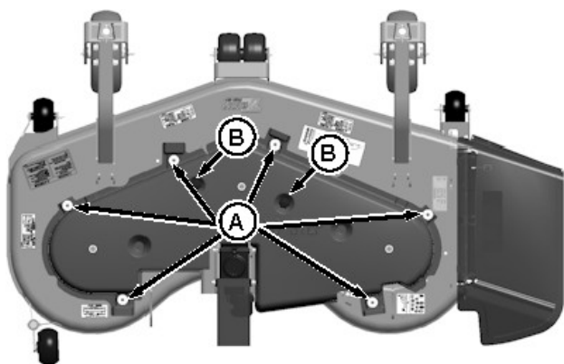
TC1011350—UN—05OCT15 Note de l'illustration: Unité de coupe à décharge latérale de 60" illustrée.
