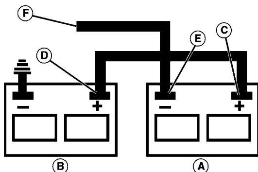
A—Akumulator pomocniczy
