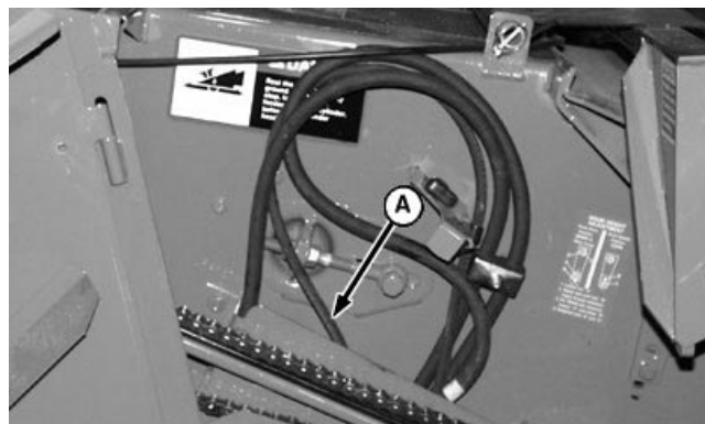
A—Mangueras hidráulicas
