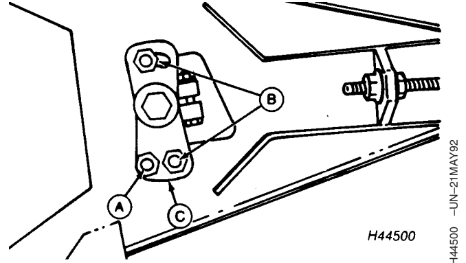
A—Perno y tuerca B—Tuercas C—Pieza de fundición
