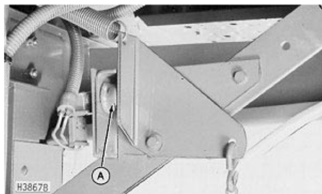
Conmutador apagado—Cosechadora 4425
