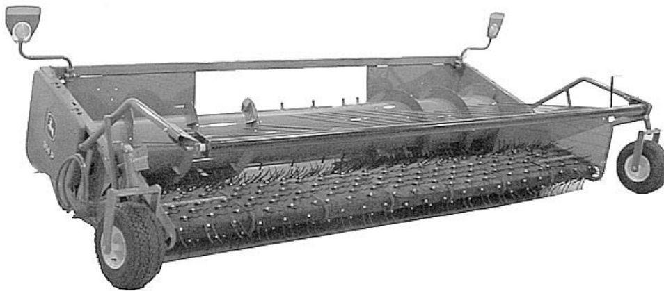
Plataforma de recolector 914 P
