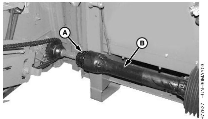
A—Acoplador de desconexión rápida B—Eje impulsor
