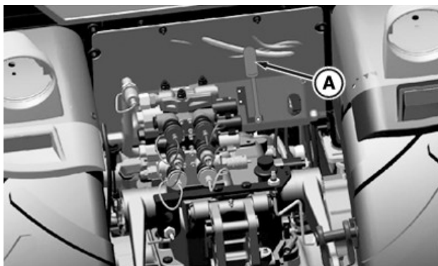
A—Atbrīvošanas svira
