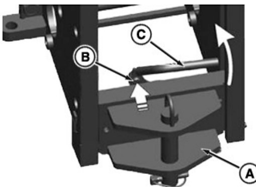
CUNA sakabe
