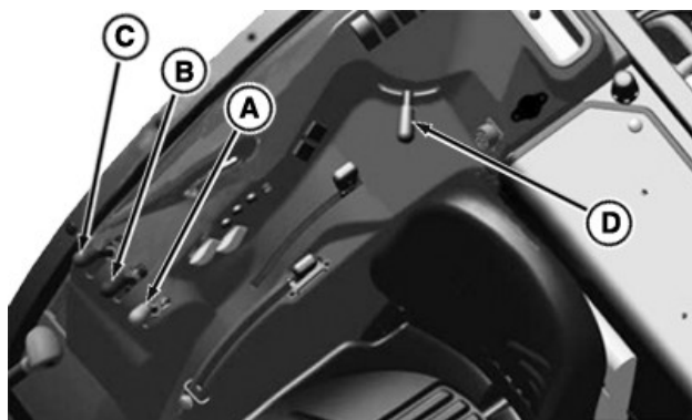
Parādīts traktors ar 4 SCV vārstiem
