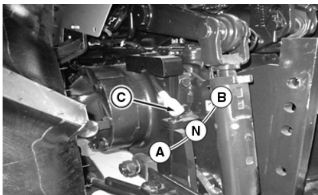
A—Jūgvārpstas apgriezieni 540 apgr./min B—Jūgvārpstas apgriezieni 540E/1000 apgr./min C—Svira N—Neitrālā pozīcija
