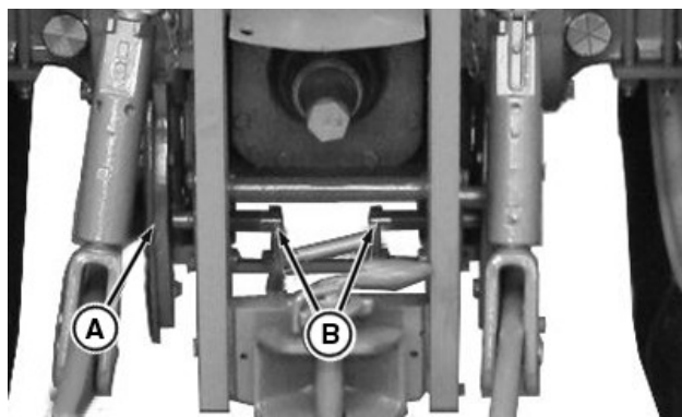
A—Šūpošanās bloki B—Skrūves
