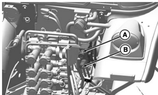
A—Savienotāji (augsta spiediena līnija) B—Savienotāji (zema spiediena līnija)
