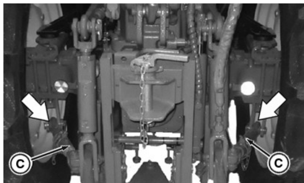
Stabilizatora stieņi
