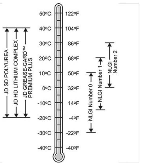
Smērvielu piemērotība gaisa temperatūru diapazoniem
