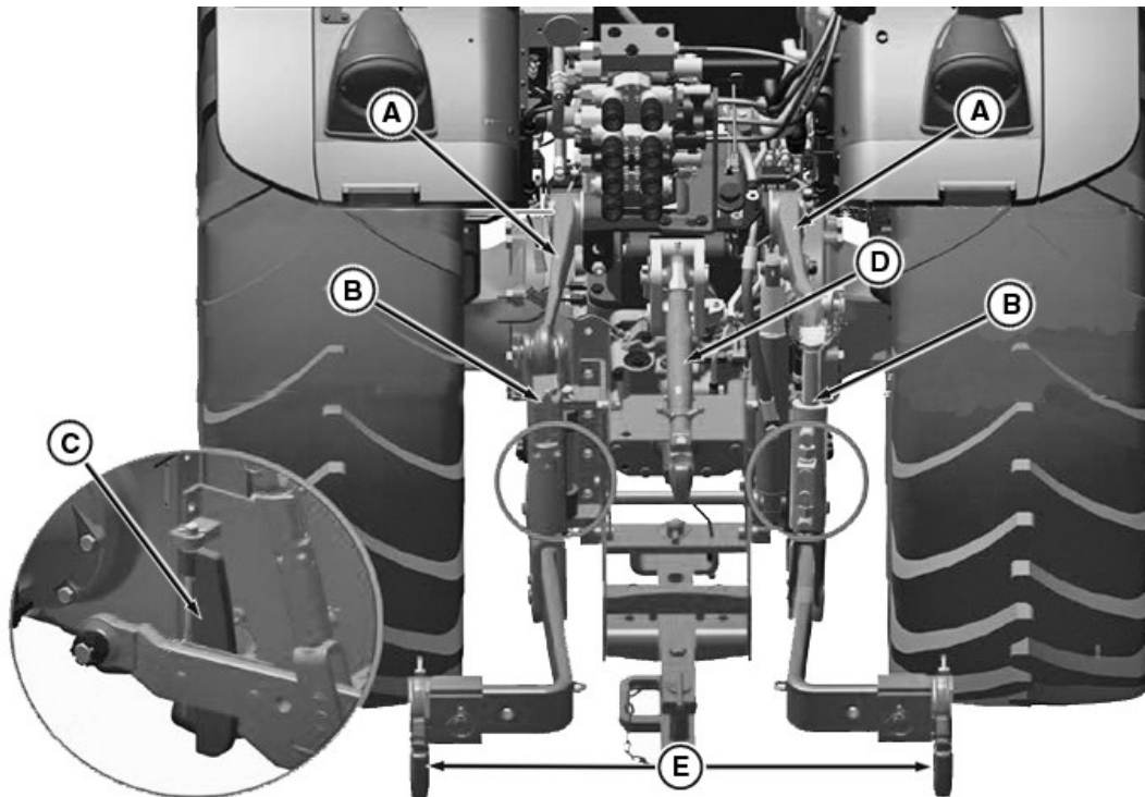
Traktors ar mehānisko stabilizācijas sistēmu
