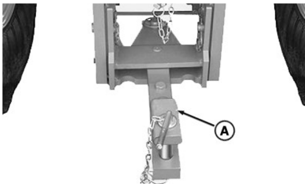
A—Jūgstienis ar vertikālu slodzi
