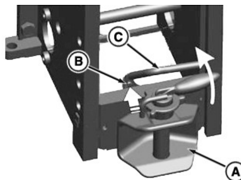
EEC sakabe
