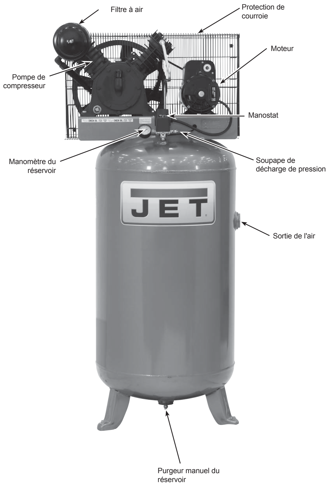
Figure 1 - Caractéristiques du compresseur
