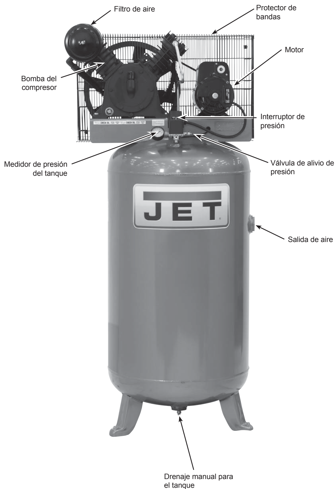
Figura 1 - Características del compresor
