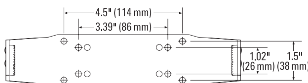
Trou Support Motif Mesures
