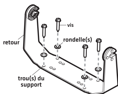
Installation du support à cardan
