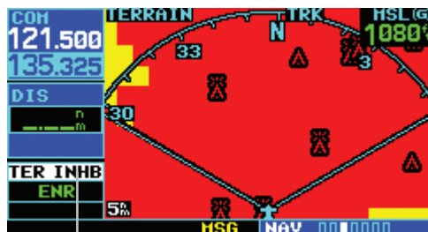
Annunciator Field
