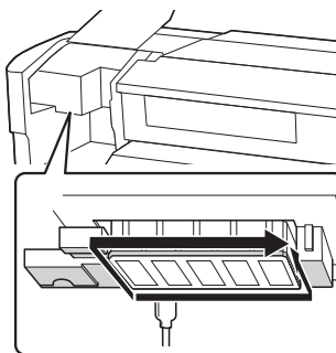
Cabezal de impresión derecho en la S30675/S50675/S70675
