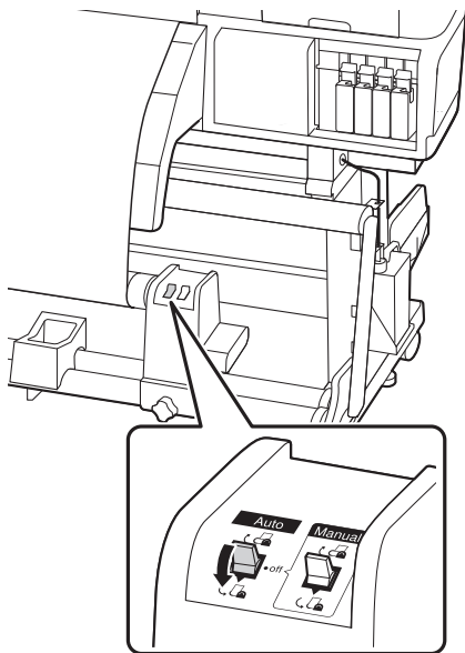
Lado impresso para fora
