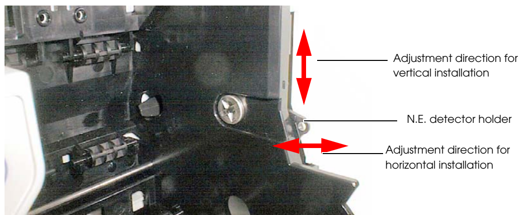
N.E. Detector Holder
