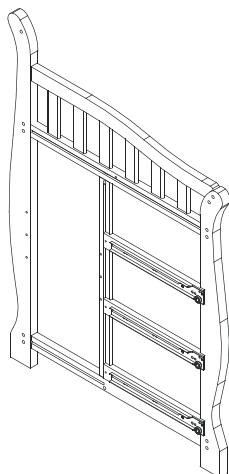
A: Changer right side (1pc) A : Côté droit de la table à langer (1pc)
