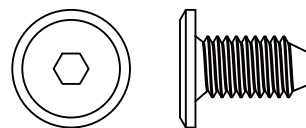
R. M8 x 15 mm Bolt x 4
