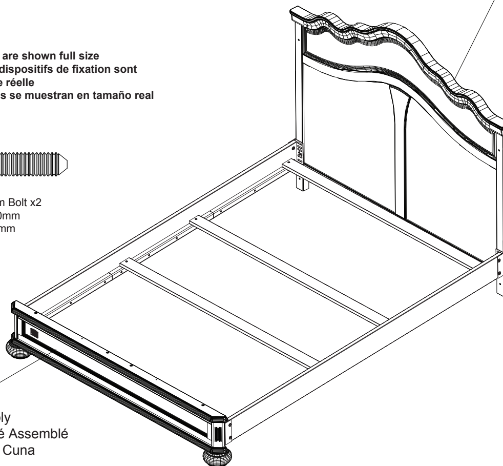
C. Back Rail x1 Panneau Arrière Barandilla Posterior
