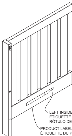
E. Left Crib Side x 1 Côté gauche du lit de bébé x 1 Costado izquierdo de la cuna x 1 25825
