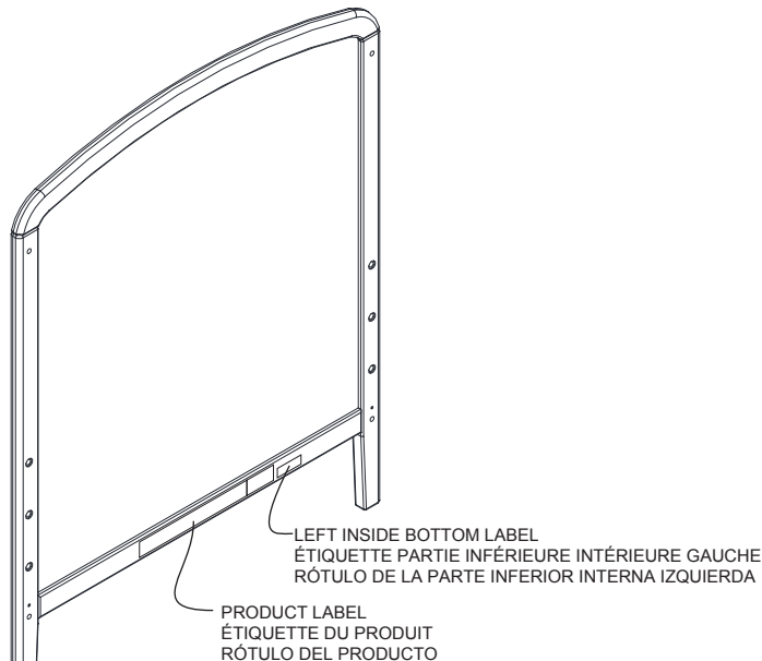
A. Left Crib End without Art x 1 Extrémité gauche du lit de bébé sans Art x 1 Extremo Izquierdo de la Cuna sin Arte x 1 27179
