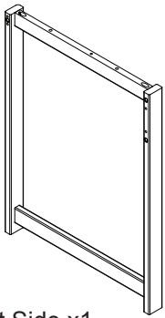
A. Left Side x1 Côté gauche Lado izquierdo # 26572
