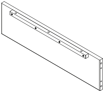
T. Left Top Back Rail x1 Barre supérieur arrière gauche Barra superior trasero izquierdo # 26578
