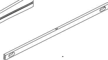
H. Bottom Back Rail x1 Barre arrière inférieur Barra trasero inferior # 26681
