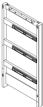
B. Right Side x1 Côté droit Lado derecho # 26674
