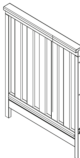
D. Right Crib Side x1 Panneau de Droite du Lit de Bébé Montaje del Lado Derecho # 26395
