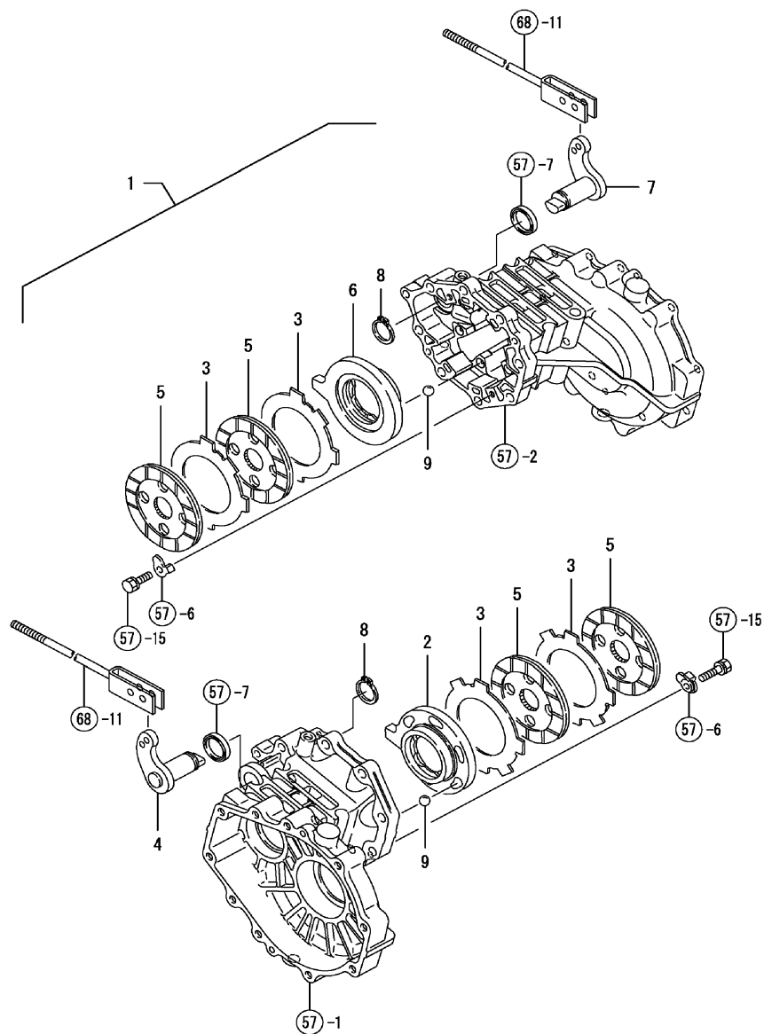
FIG. 67. DISC BRAKE
