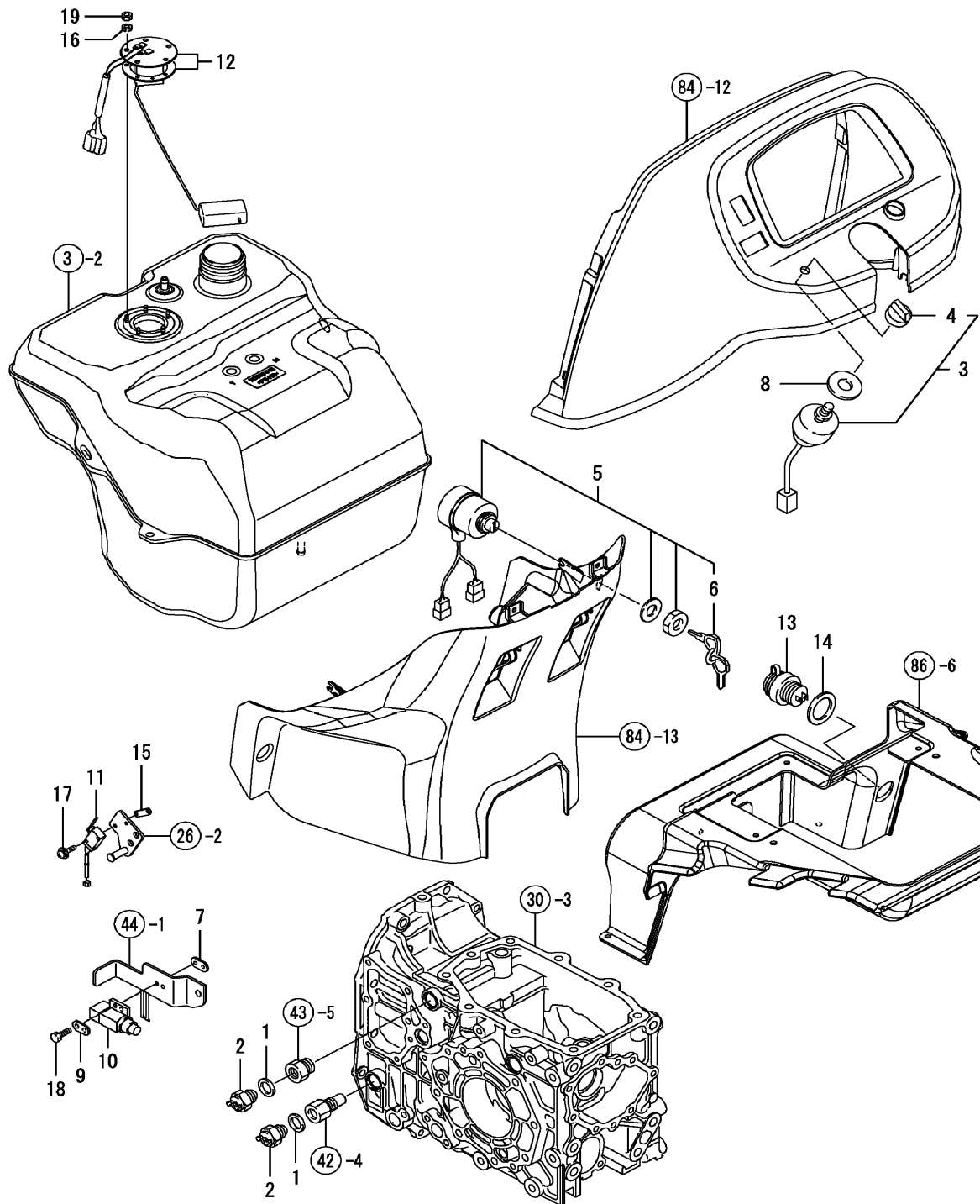
FIG. 78. SWITCH 1
