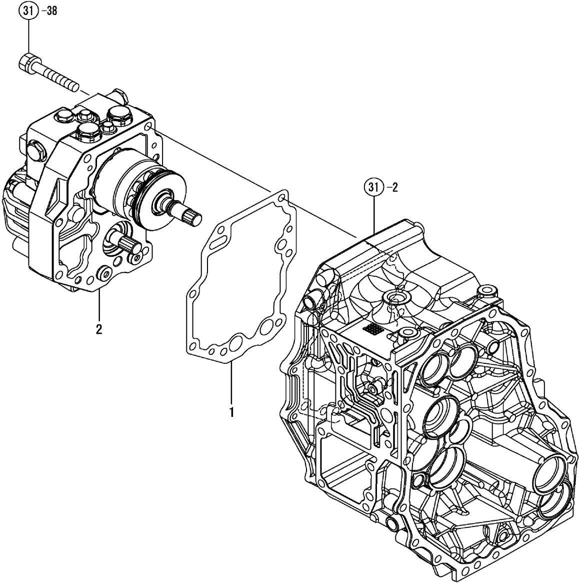
FIG. 48. H.S.T.
