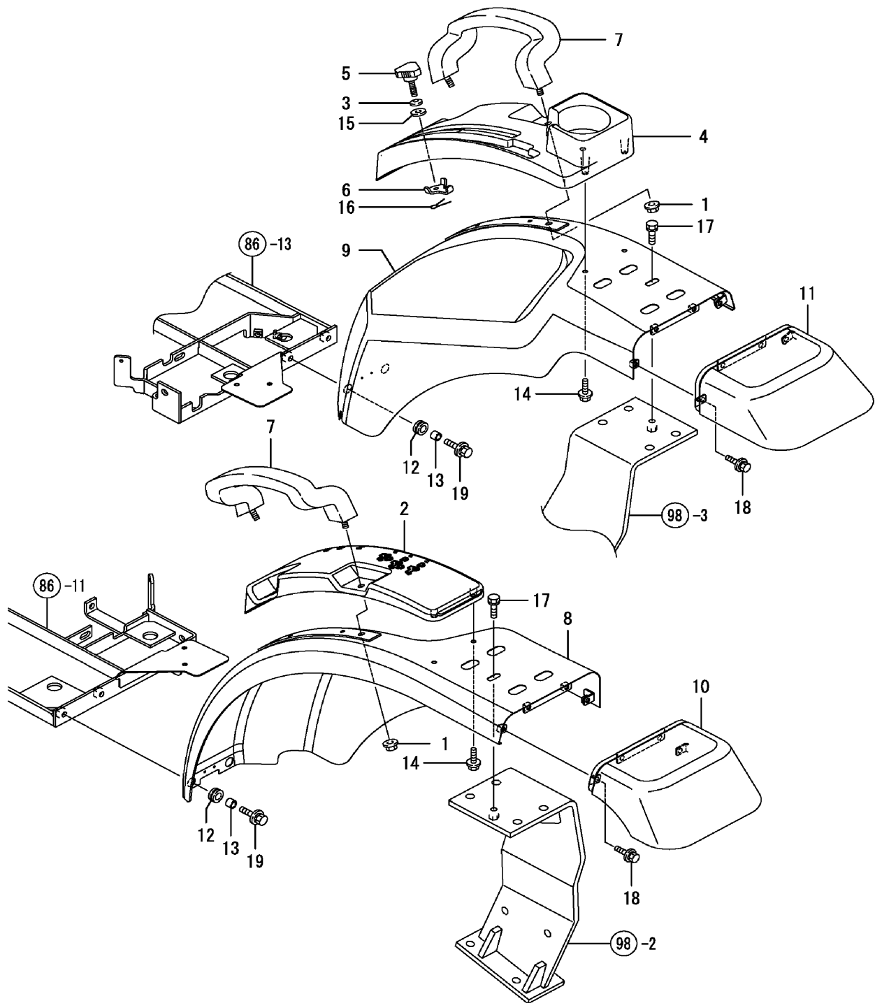
FIG. 85. FENDER
