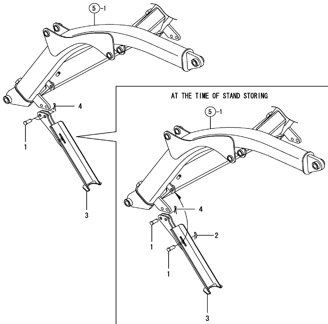
FIG. 10. STAND
