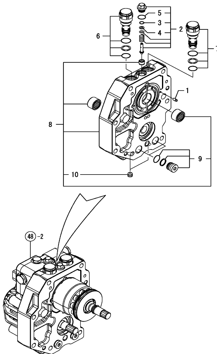
FIG. 49. CENTER CASE
