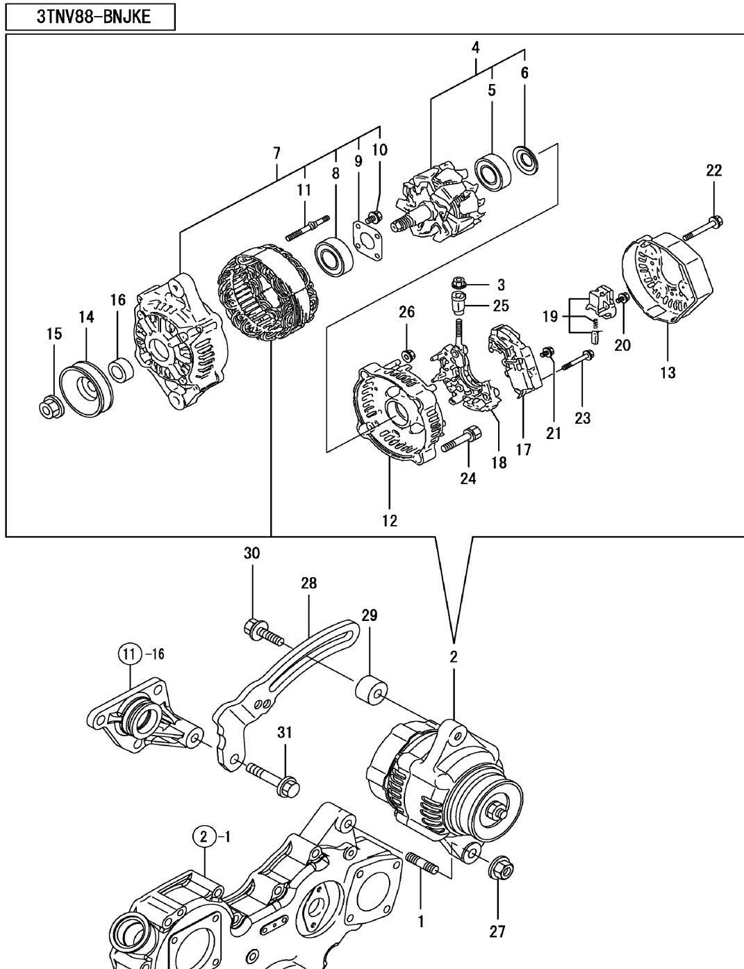
FIG. 17. GENERATOR
