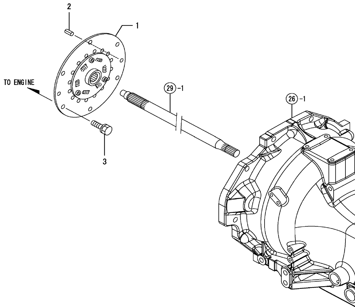
FIG. 28. DAMPER DISC
