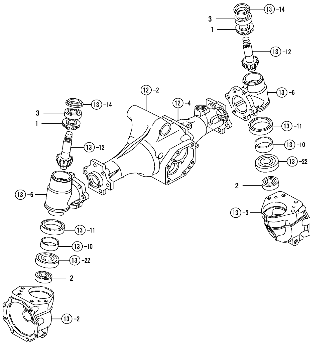
FIG. 14. FRONT SHAFT 2
