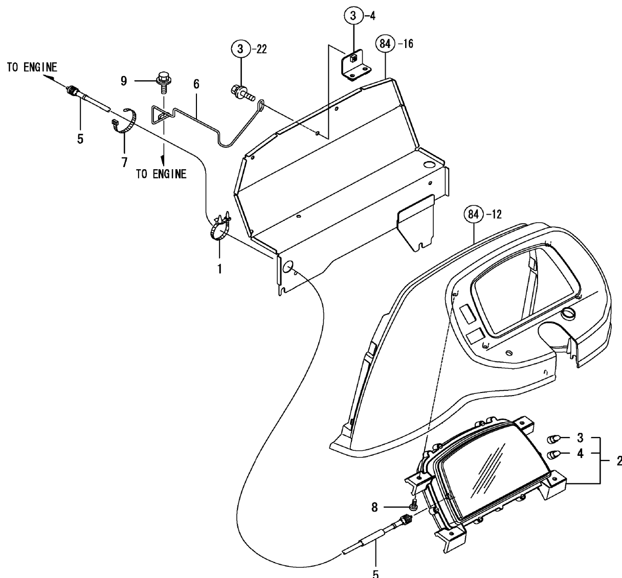
FIG. 81. METER
