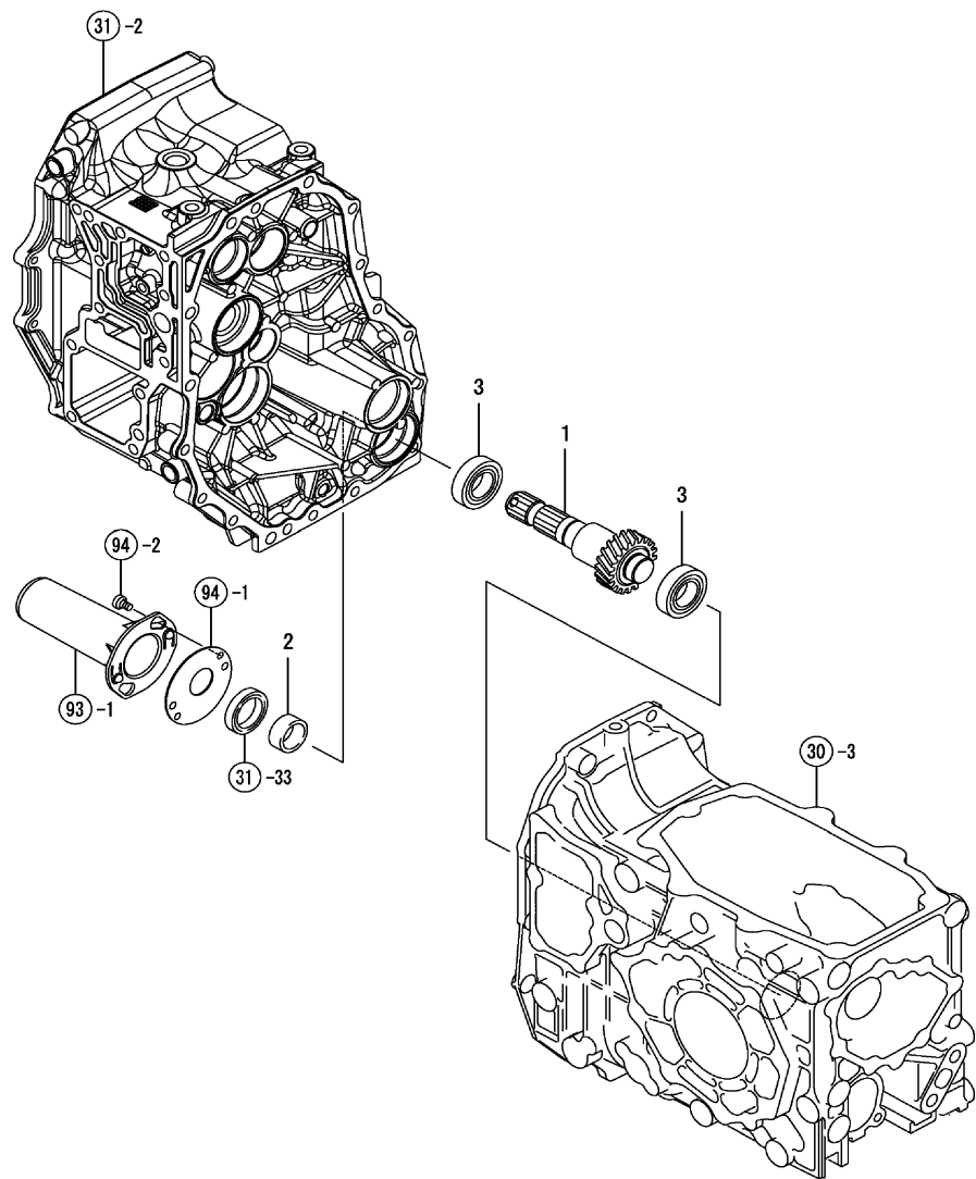
FIG. 40. MID PTO SHAFT
