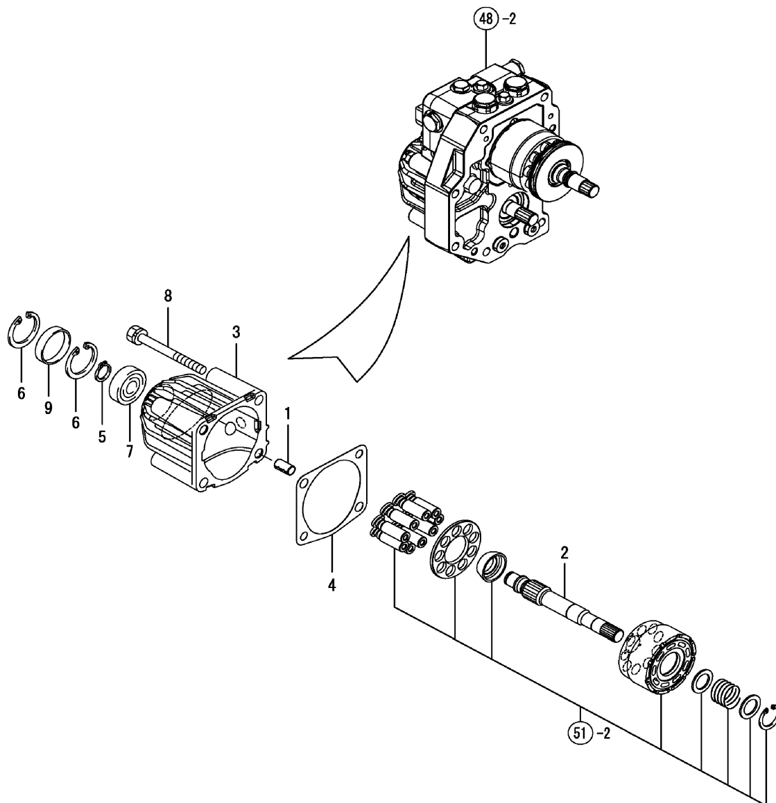
FIG. 53. MOTOR CASE
