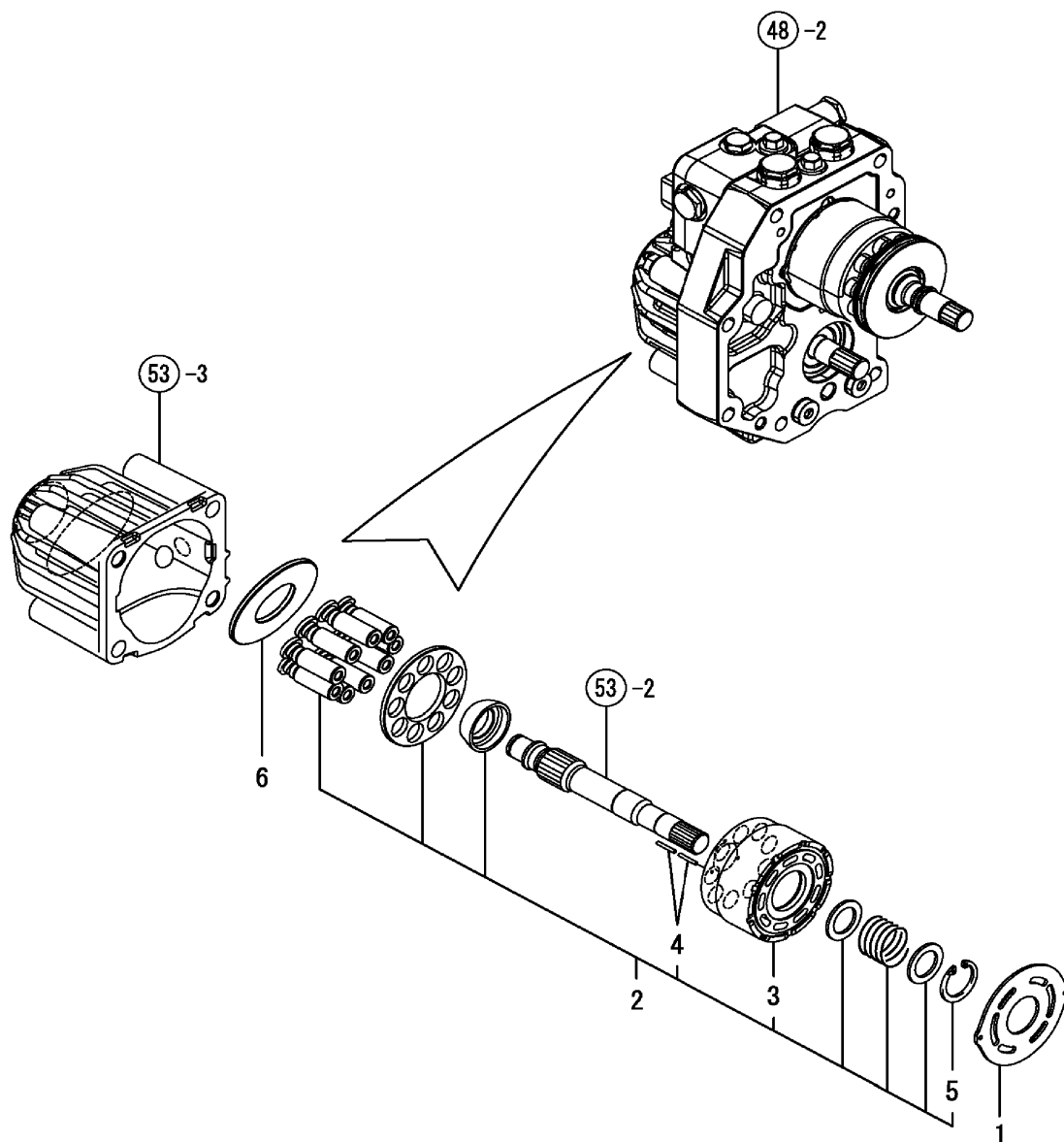
FIG. 51. MOTOR
