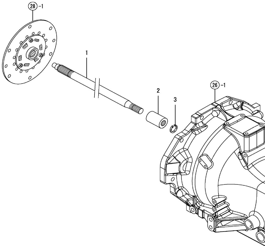
FIG. 29. CLUTCH SHAFT
