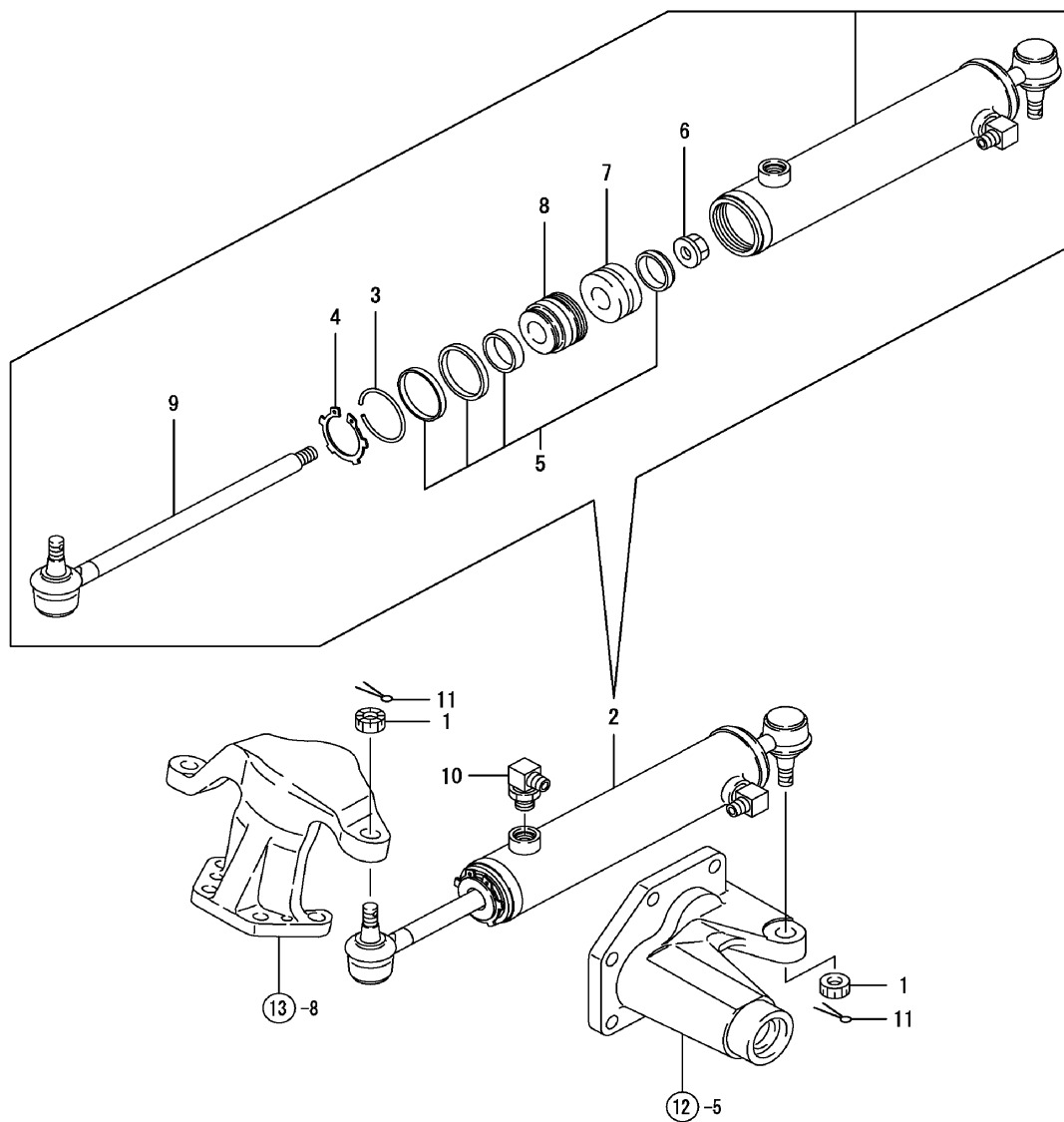
FIG. 23. PST CYLINDER
