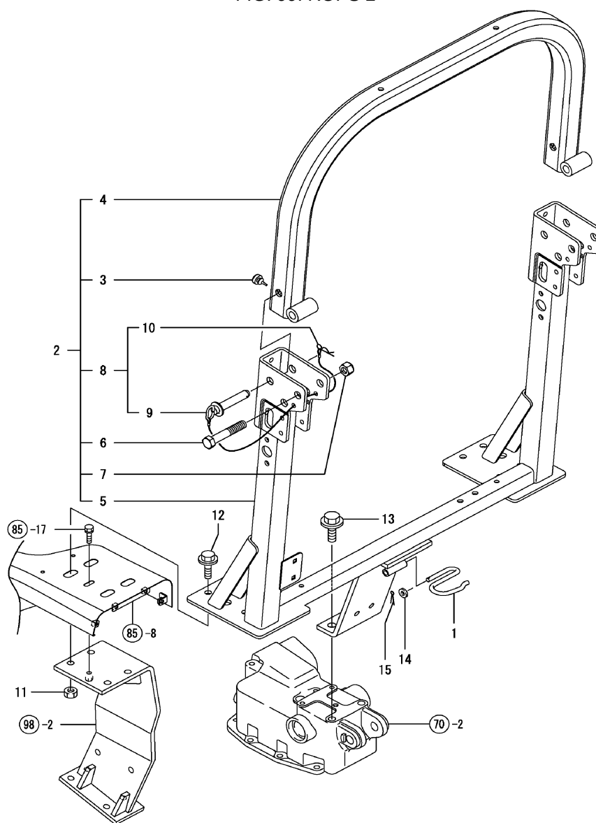
FIG. 99. ROPS 2
