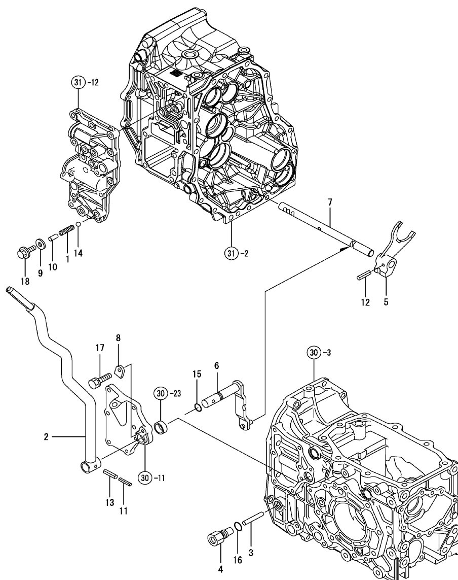
FIG. 42. RANGE SHIFT
