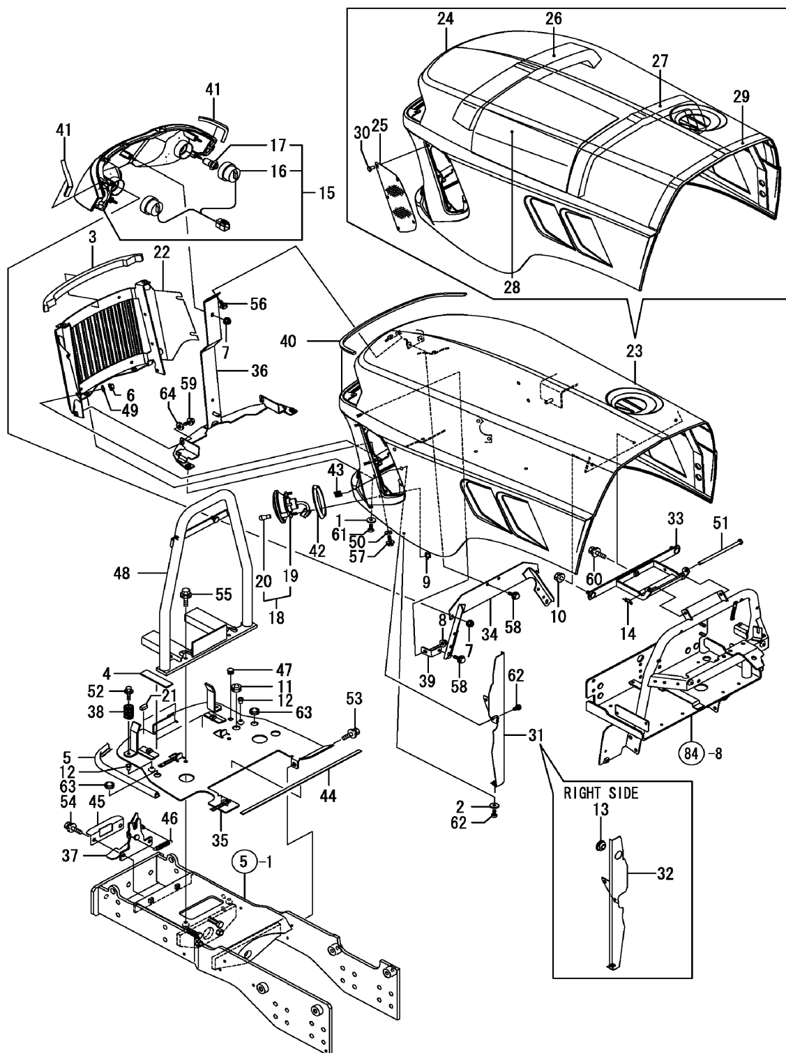
FIG. 83. HOOD
