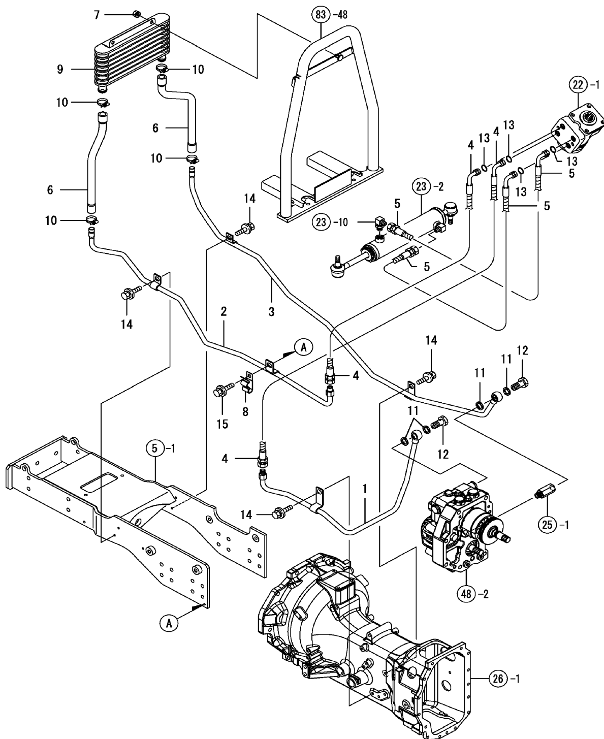
FIG. 24. PST PIPING A
