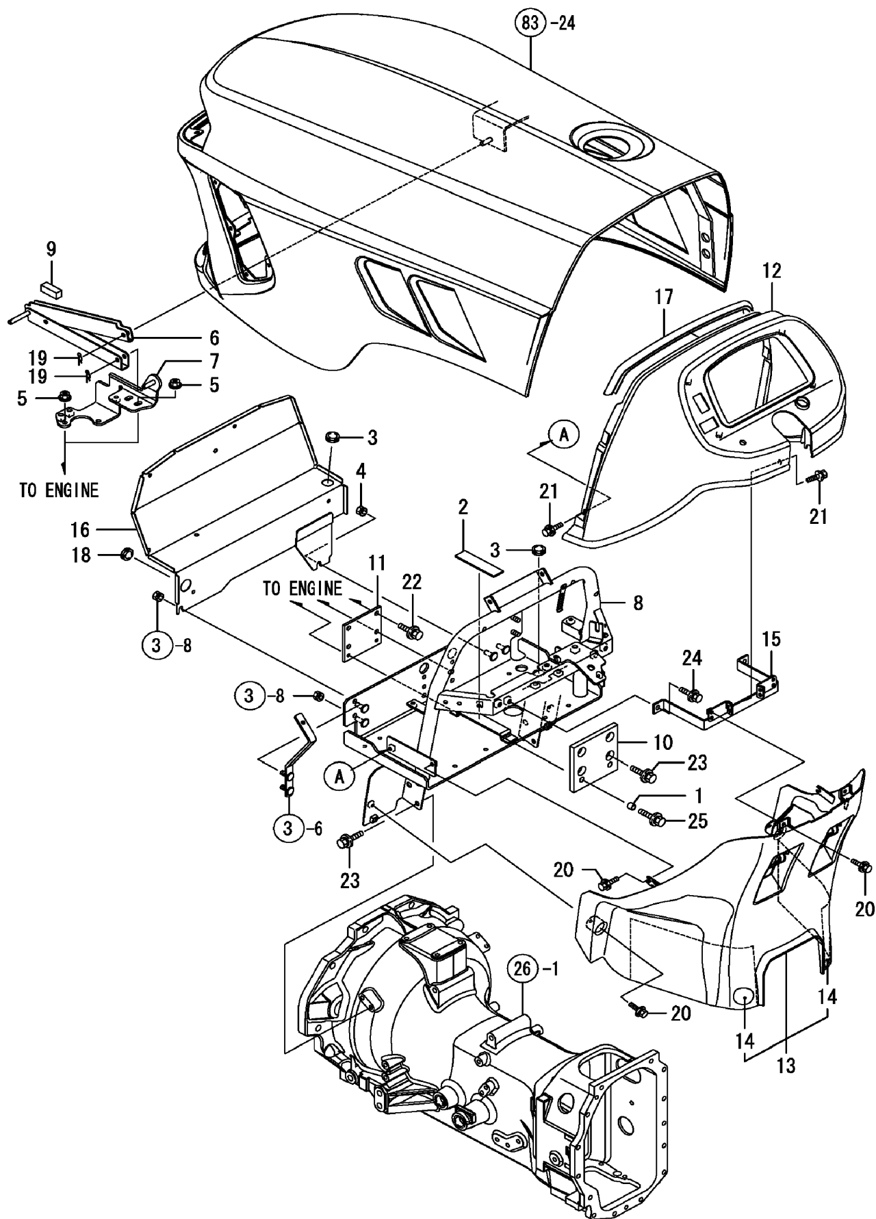
FIG. 84. DASHBOARD
