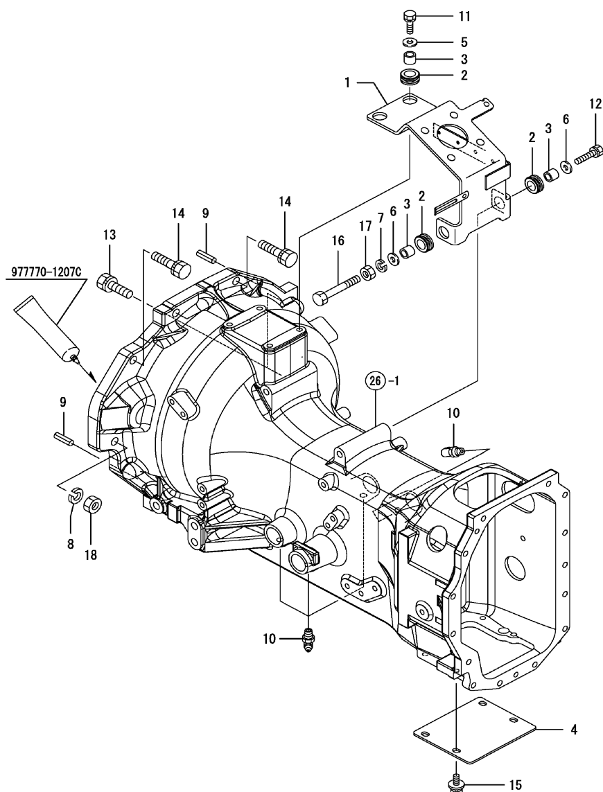
FIG. 27. DOCKING BOLT
