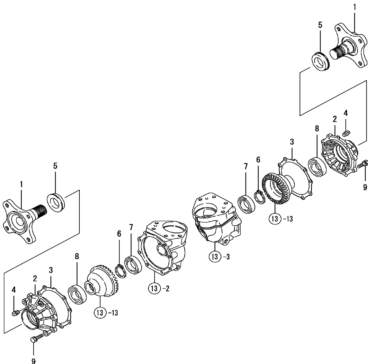
FIG. 16. FRONT SPINDLE
