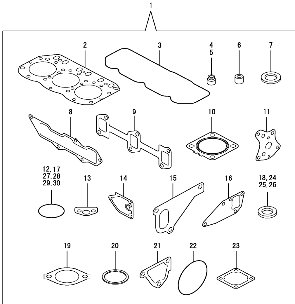
FIG. 18. GASKET KIT
