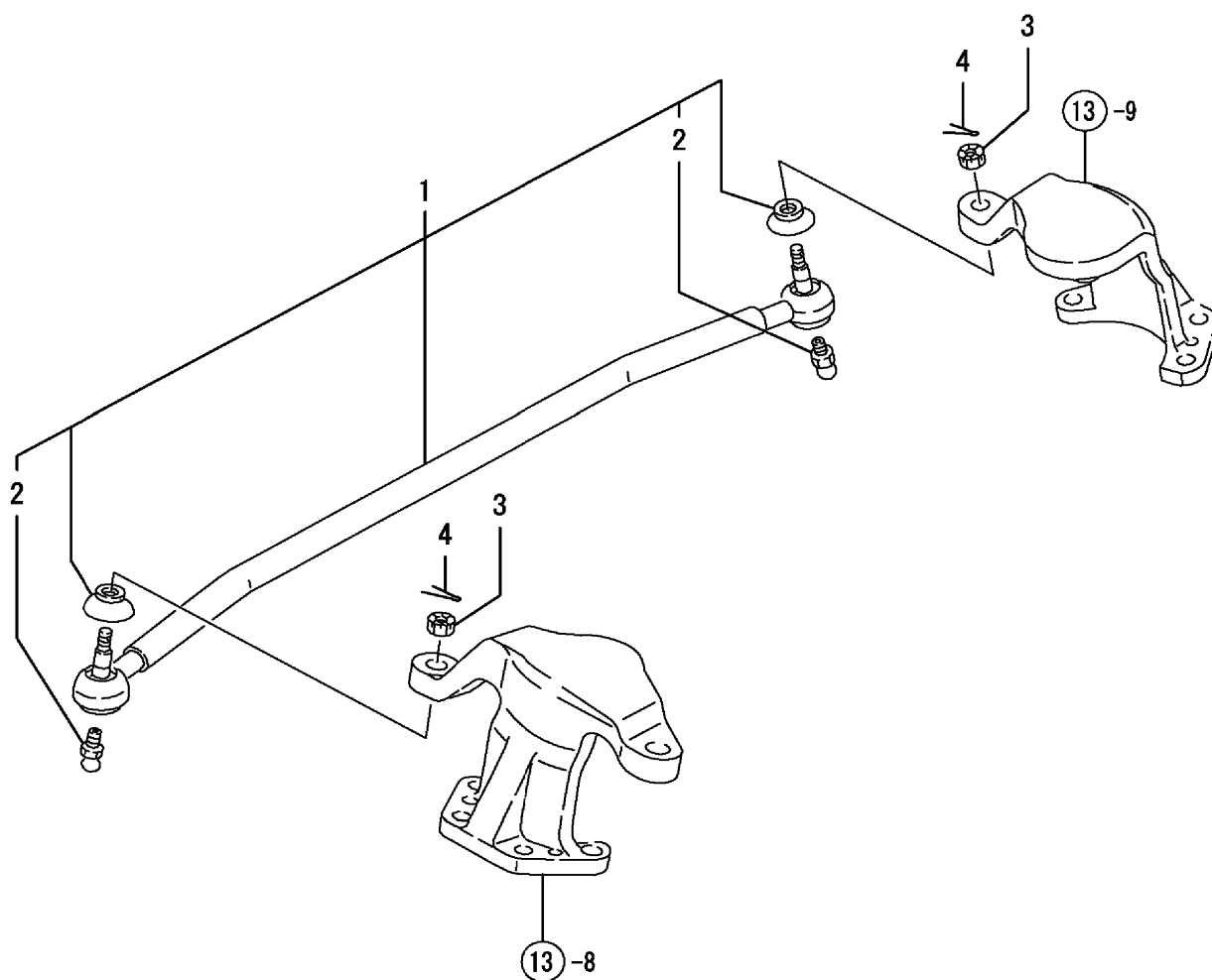
FIG. 7. TIE-ROD
