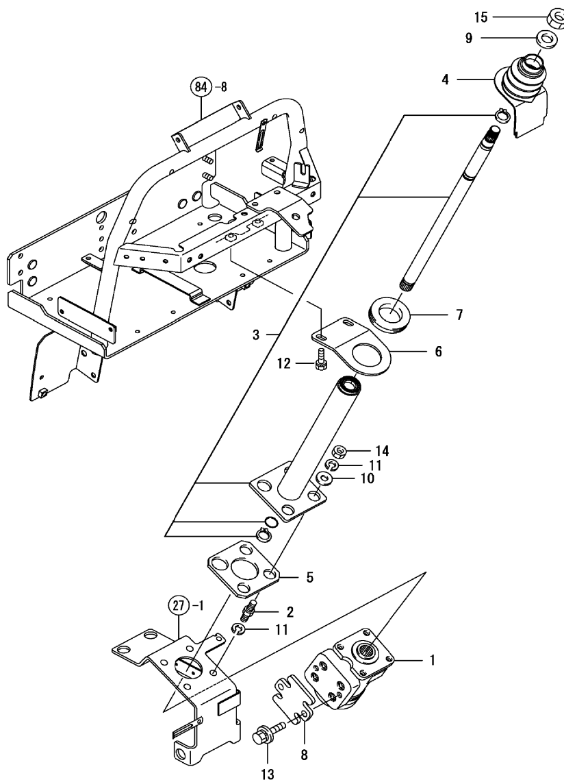
FIG. 22. PST VALVE
