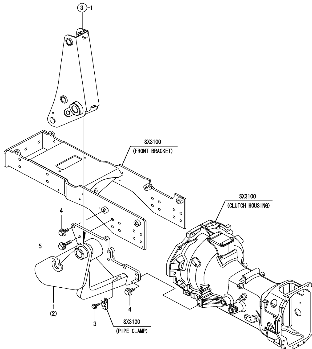
FIG. 4. BRACKET
