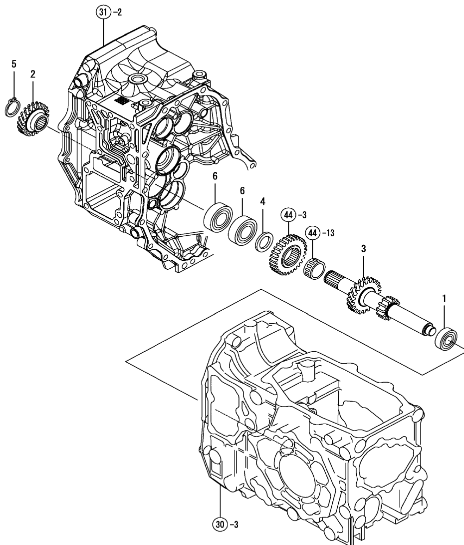
FIG. 35. MAIN SHAFT
