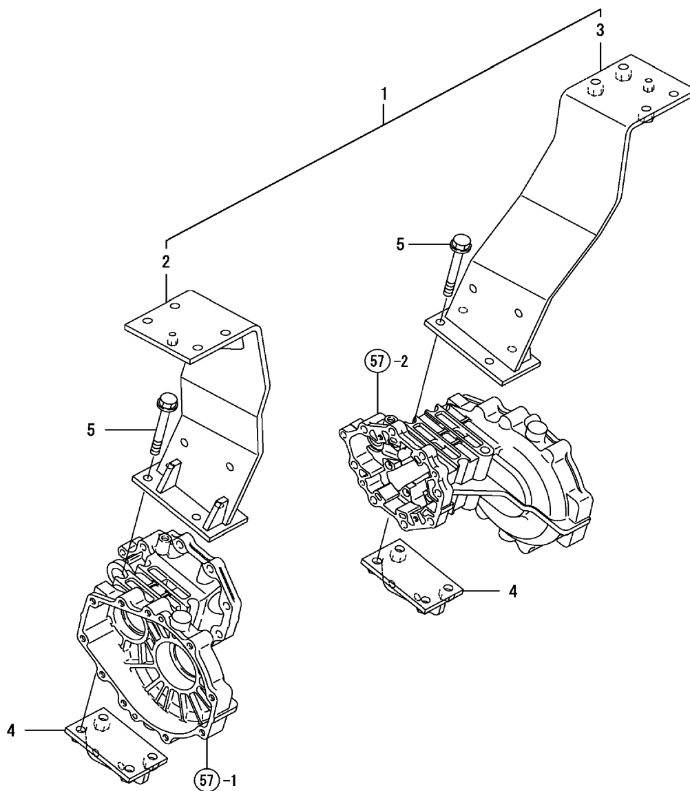
FIG. 98. ROPS 1
