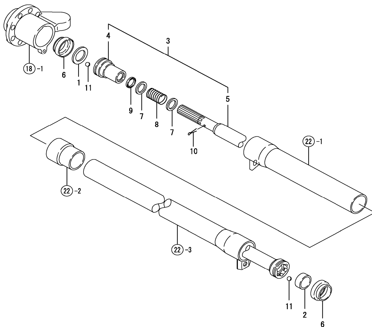
FIG. 16. PROPELLER SHAFT
