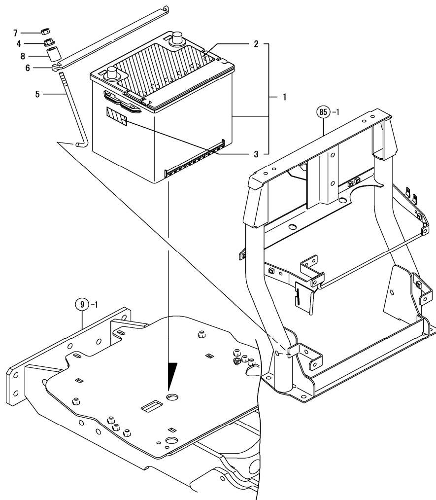
FIG. 78. BATTERY
