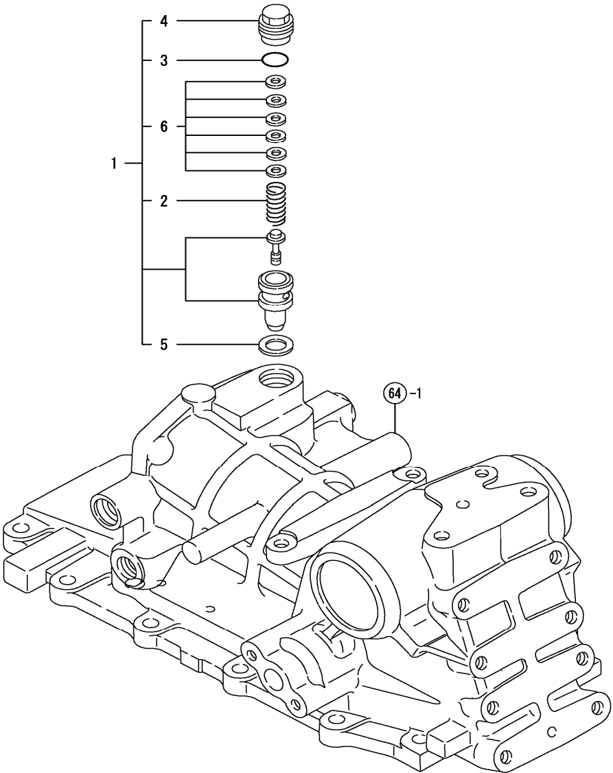
FIG. 67. RELIEF VALVE
