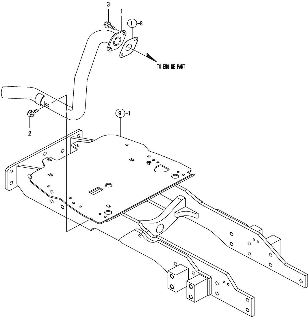
FIG. 4. EXHAUST
