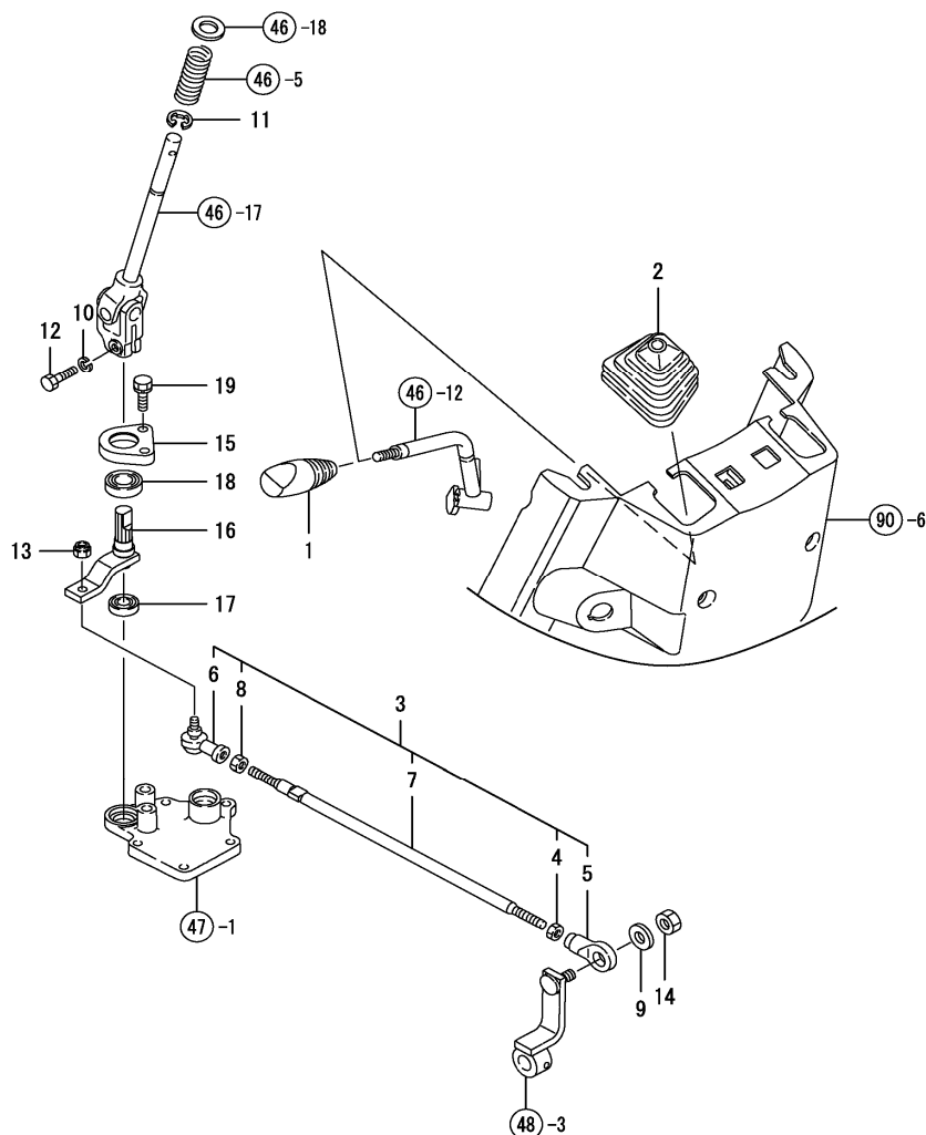
FIG. 49. REVERSE LEVER
