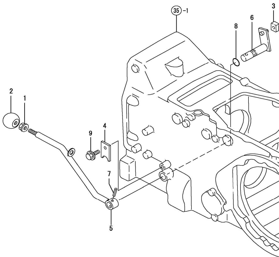
FIG. 53. FRONT SHIFT
