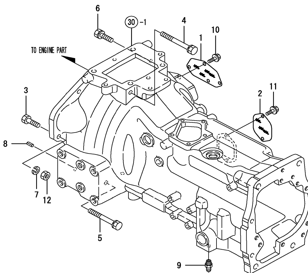
FIG. 31. DOCKING BOLT
