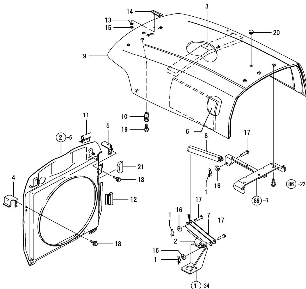
FIG. 87. HOOD
