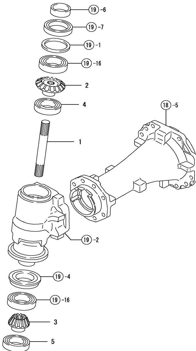
FIG. 20. FRONT SHAFT
