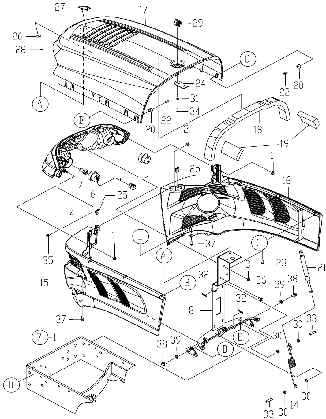
FIG. 84. HOOD
