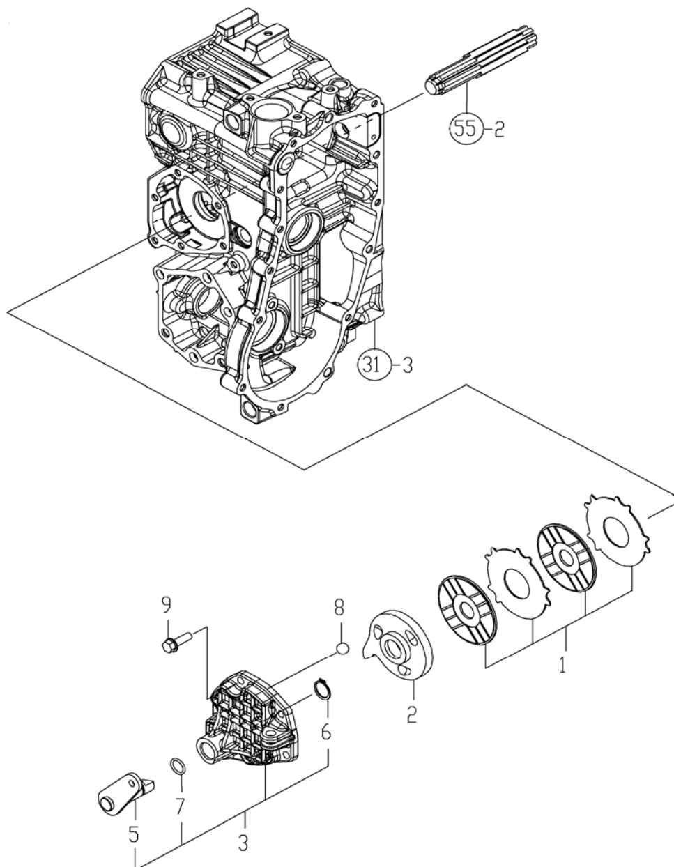
FIG. 64. DISC BRAKE
