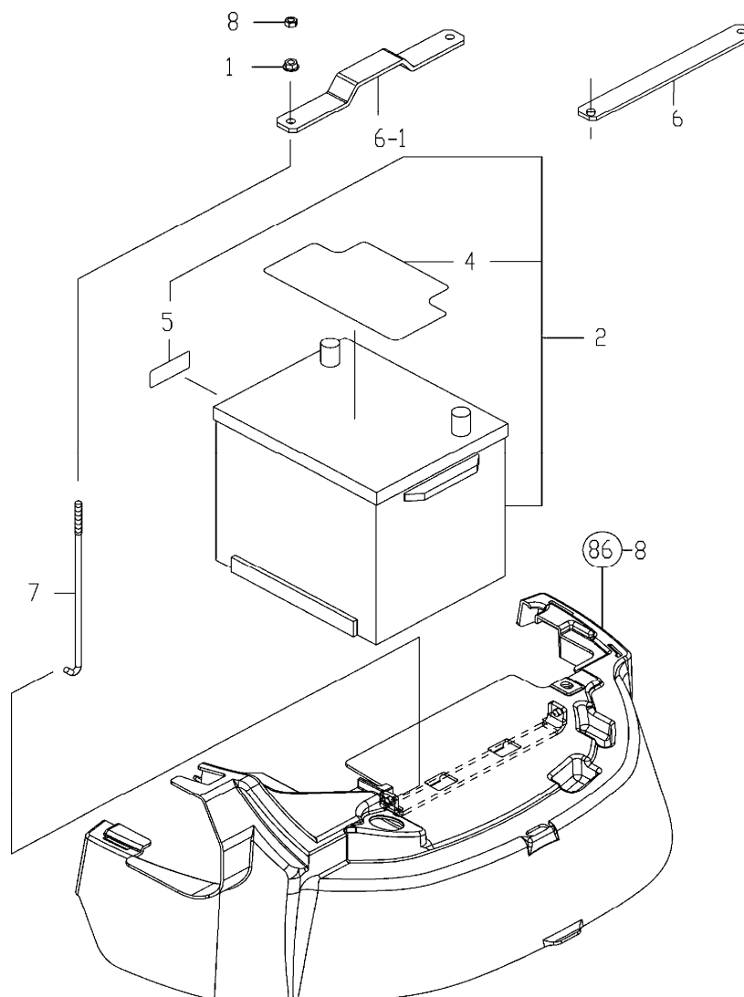
FIG. 78. BATTERY
