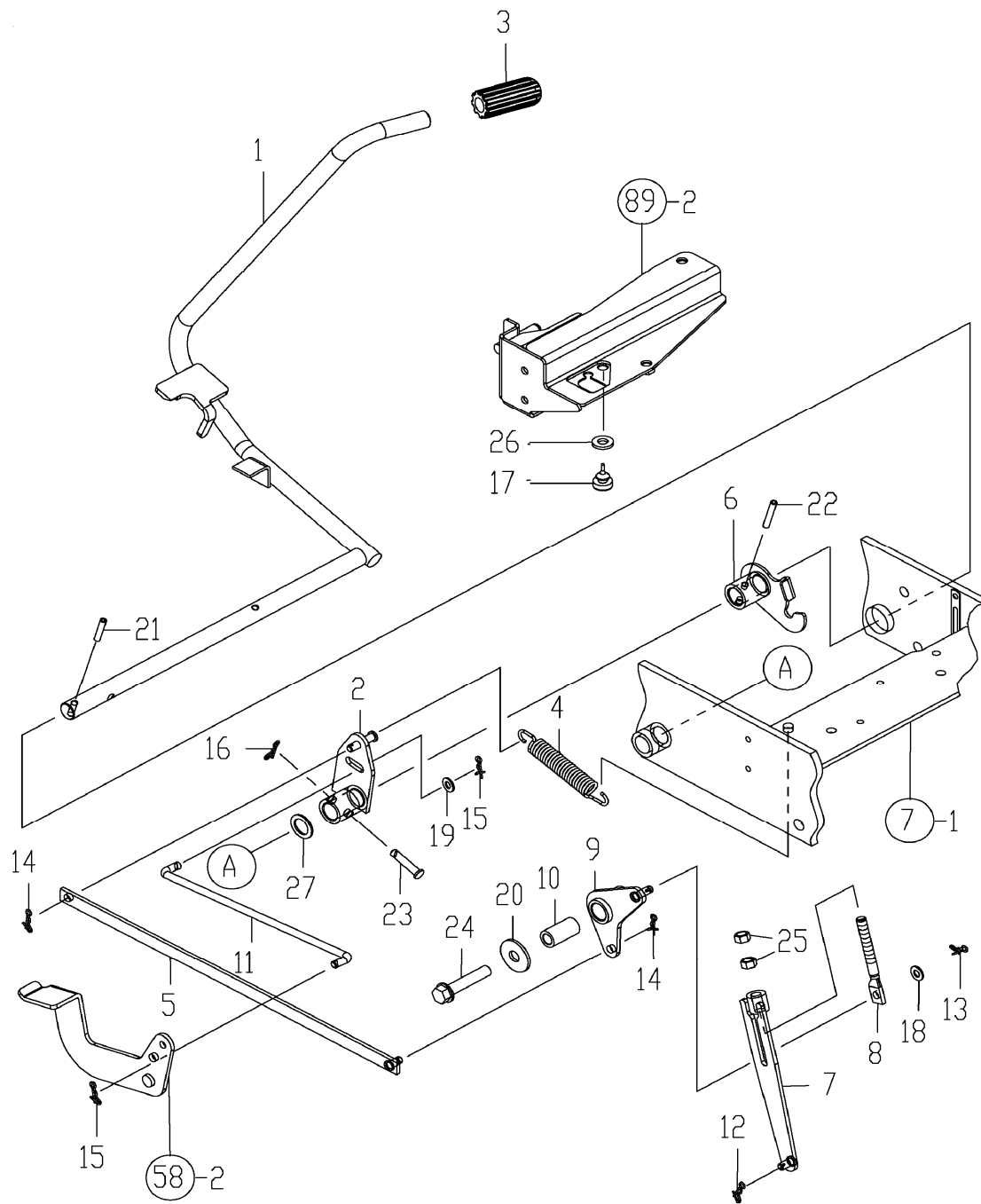
FIG. 65. BRAKE PEDAL
