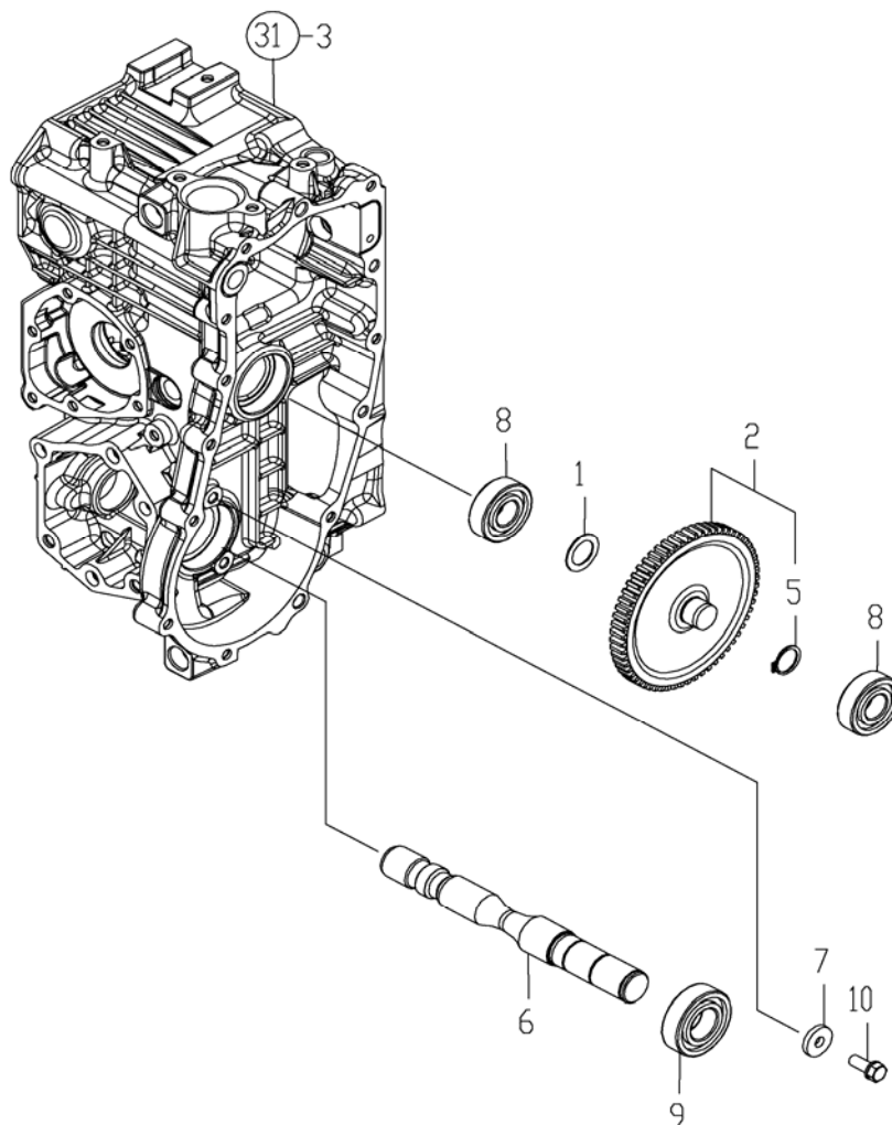
FIG. 39. P.T.O. SHAFT
