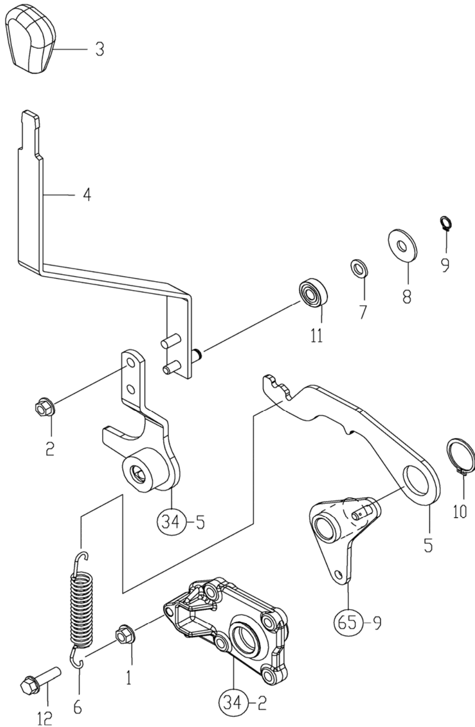
FIG. 44. RANGE LEVER
