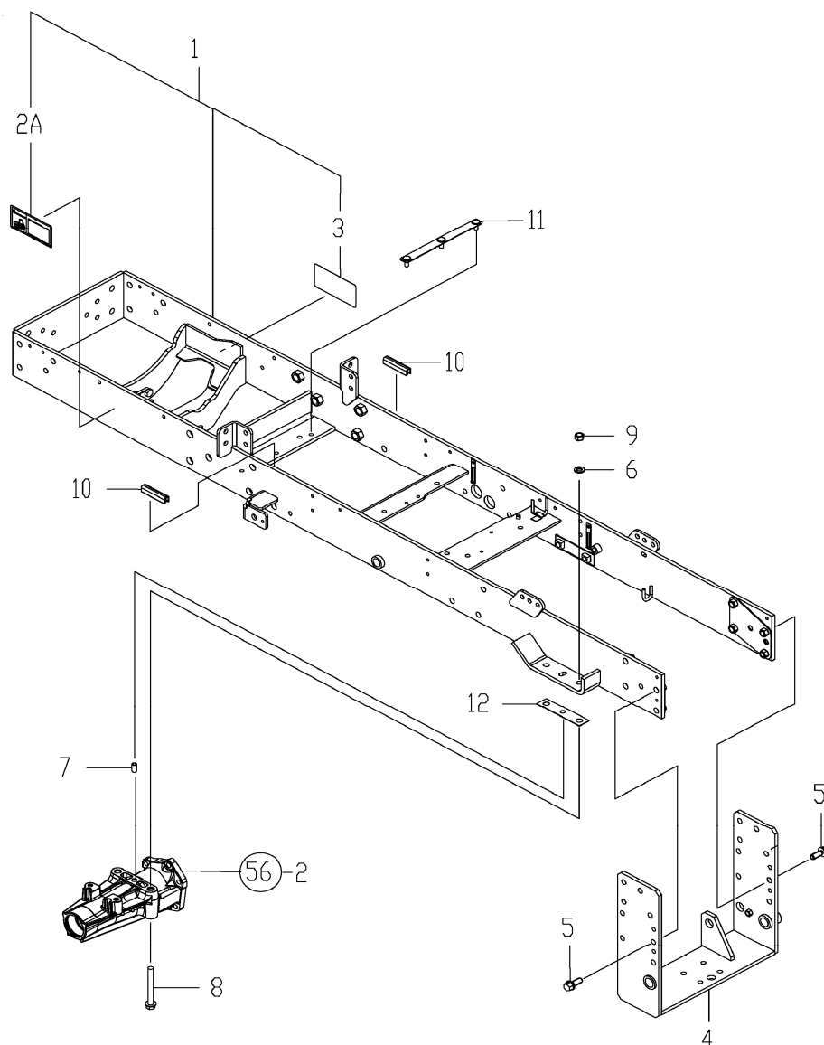
FIG. 7. FRAME
