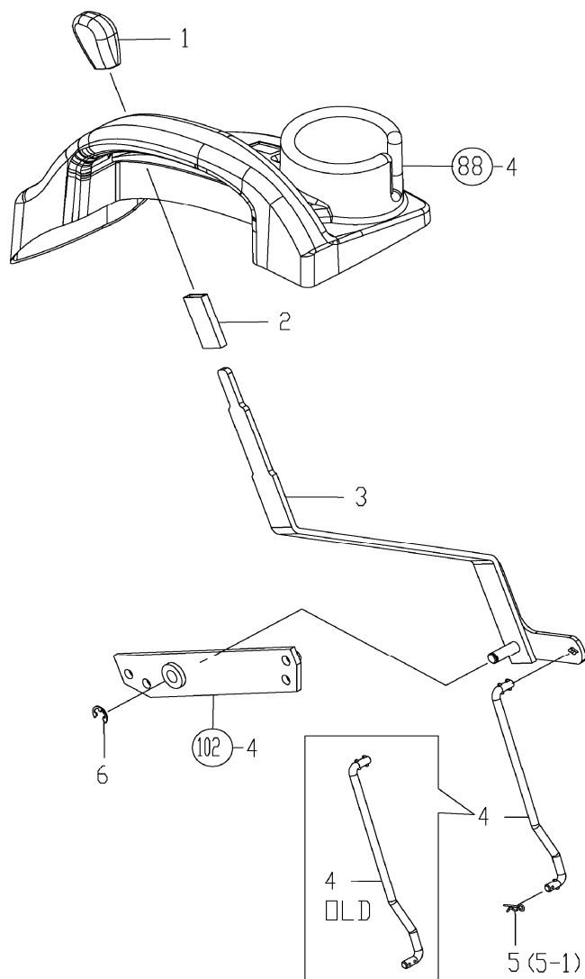
FIG. 46. P.T.O. LEVER
