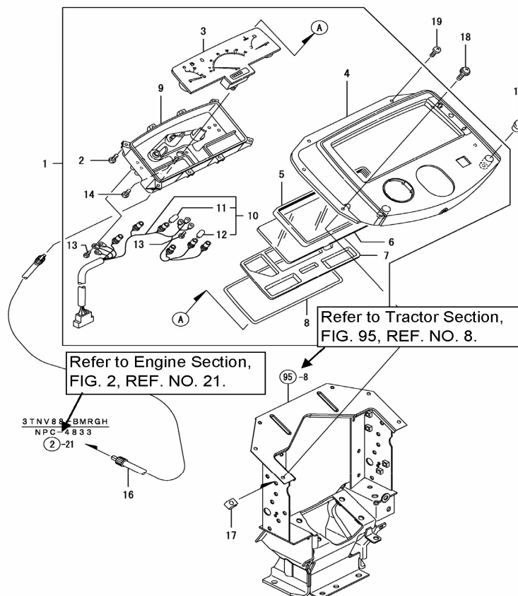
FIG. 88. METER
