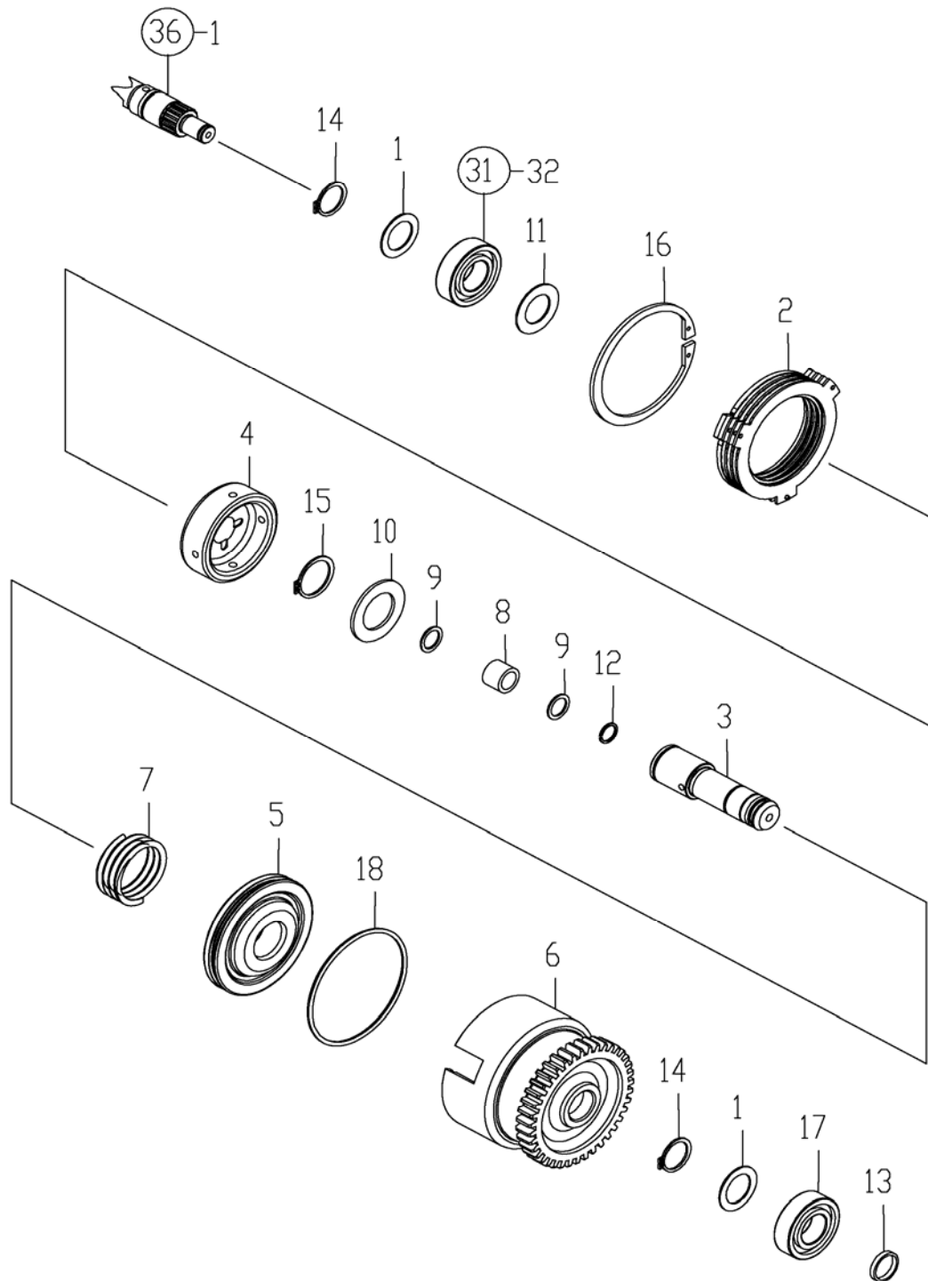
FIG. 37. CLUTCH SHAFT
