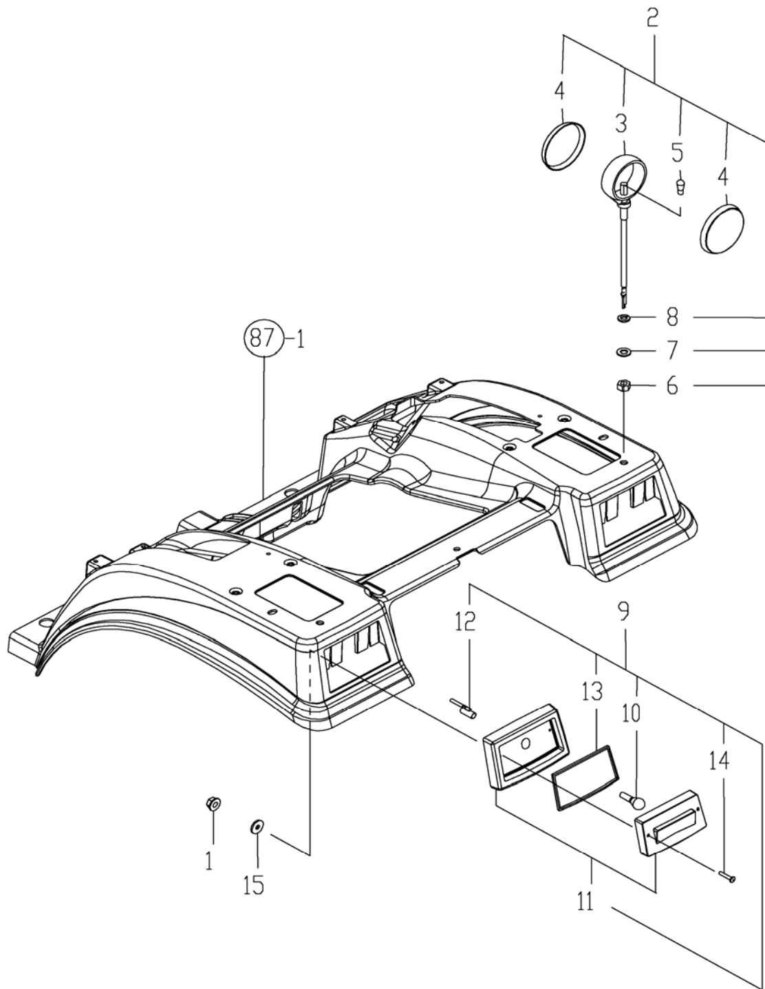
FIG. 81. LAMPS
