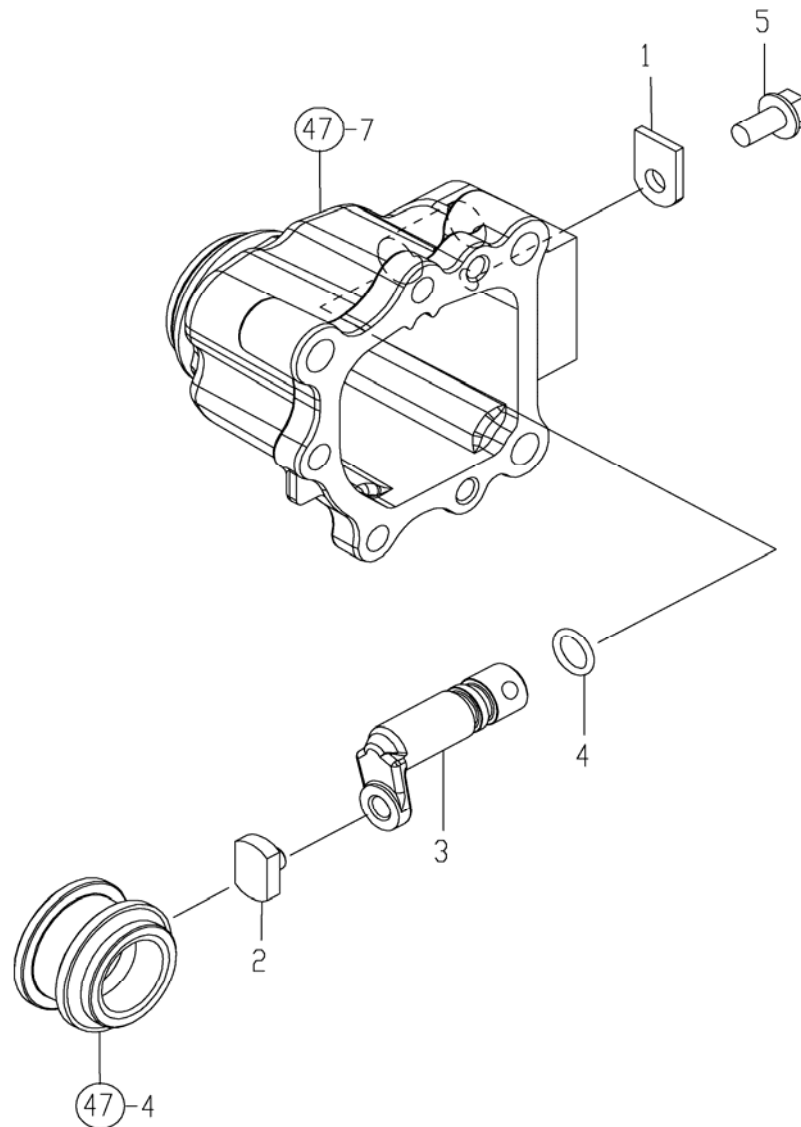
FIG. 49. MFWD SHIFT
