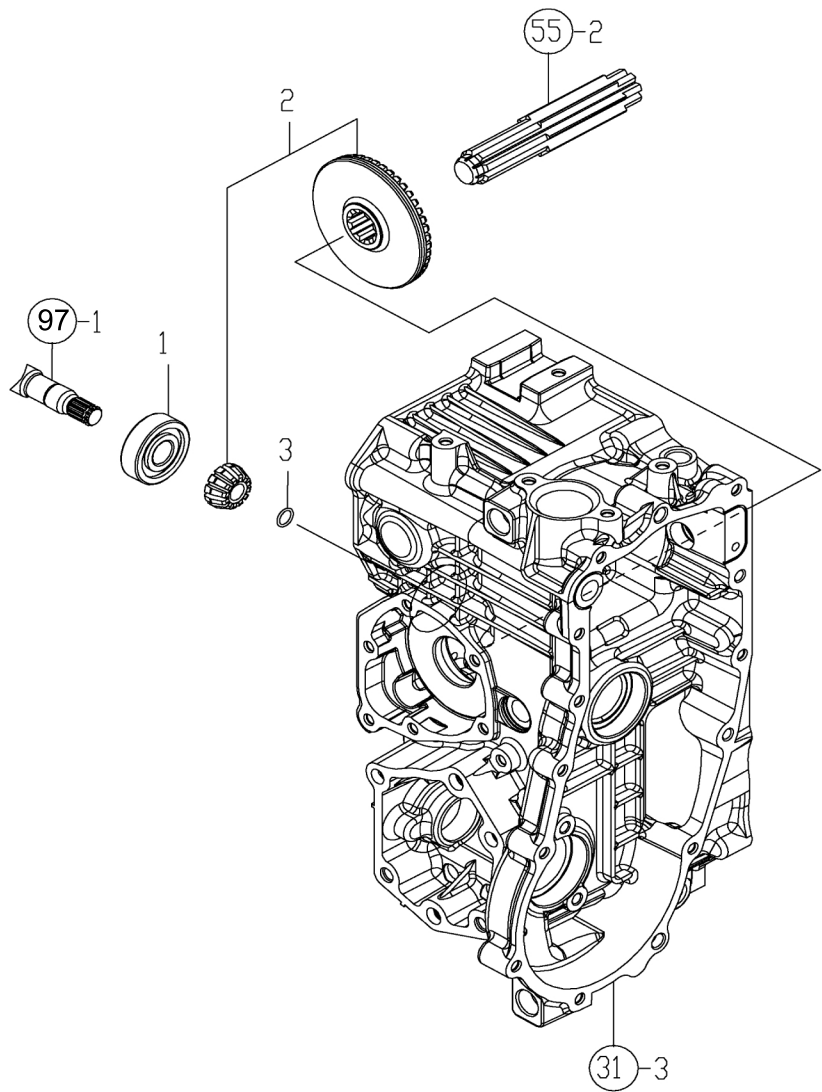
FIG. 54. INPUT GEAR
