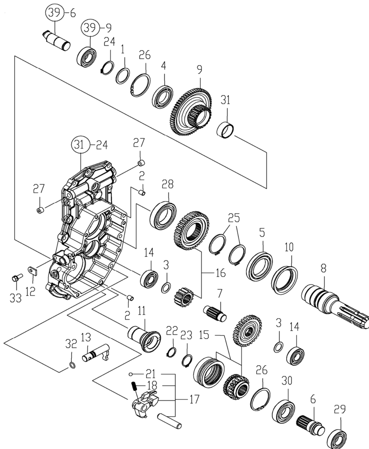
FIG. 42. REAR P.T.O. SHAFT
