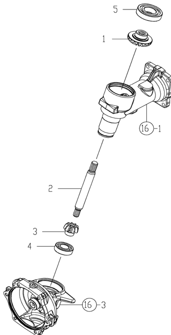
FIG. 17. FRONT SHAFT
