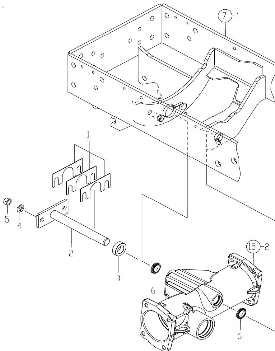
FIG. 9. CENTER PIN
