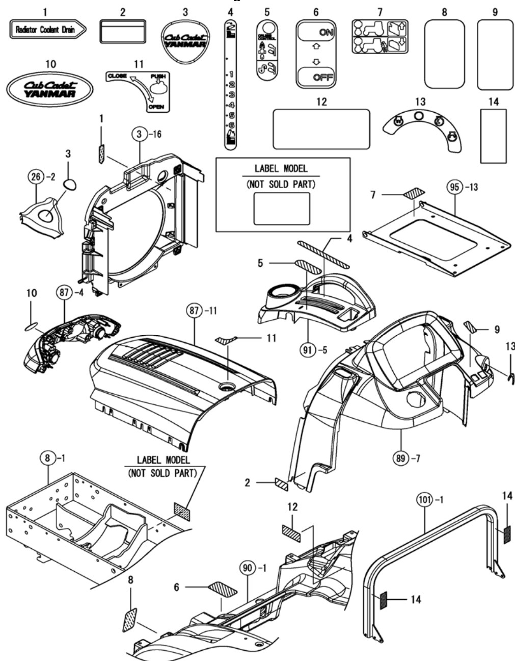
Fig. 96 - Label
