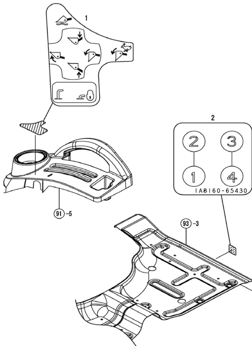
Fig. 98 - Label, SCV
