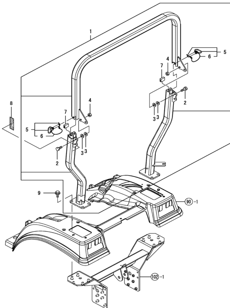
Fig. 101 - Rops Upper
