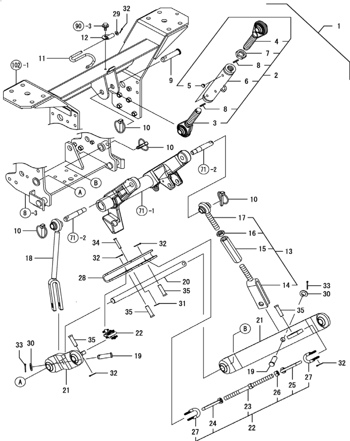
Fig. 106 - 3P Kit
