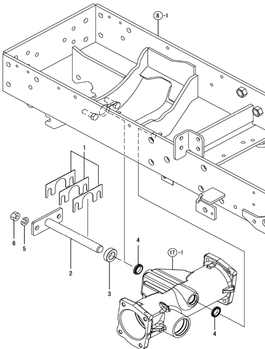
Fig. 11 - Center Pin
