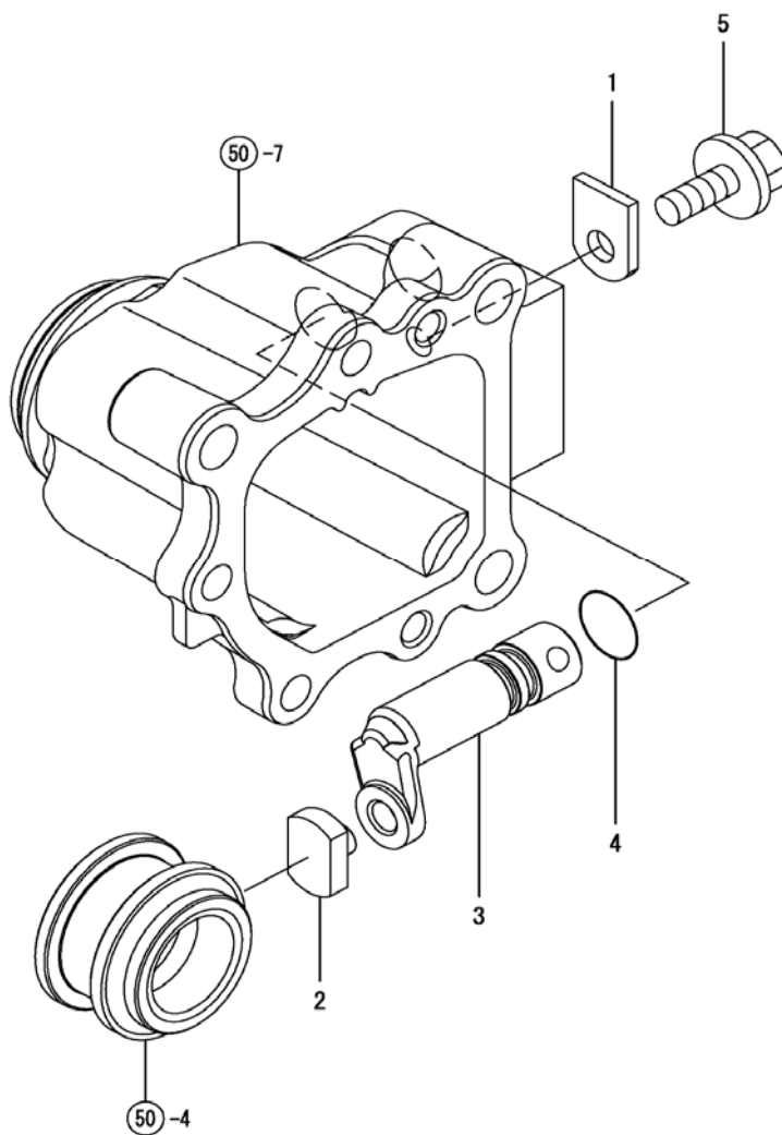
Fig. 52 - MFWD Shift
