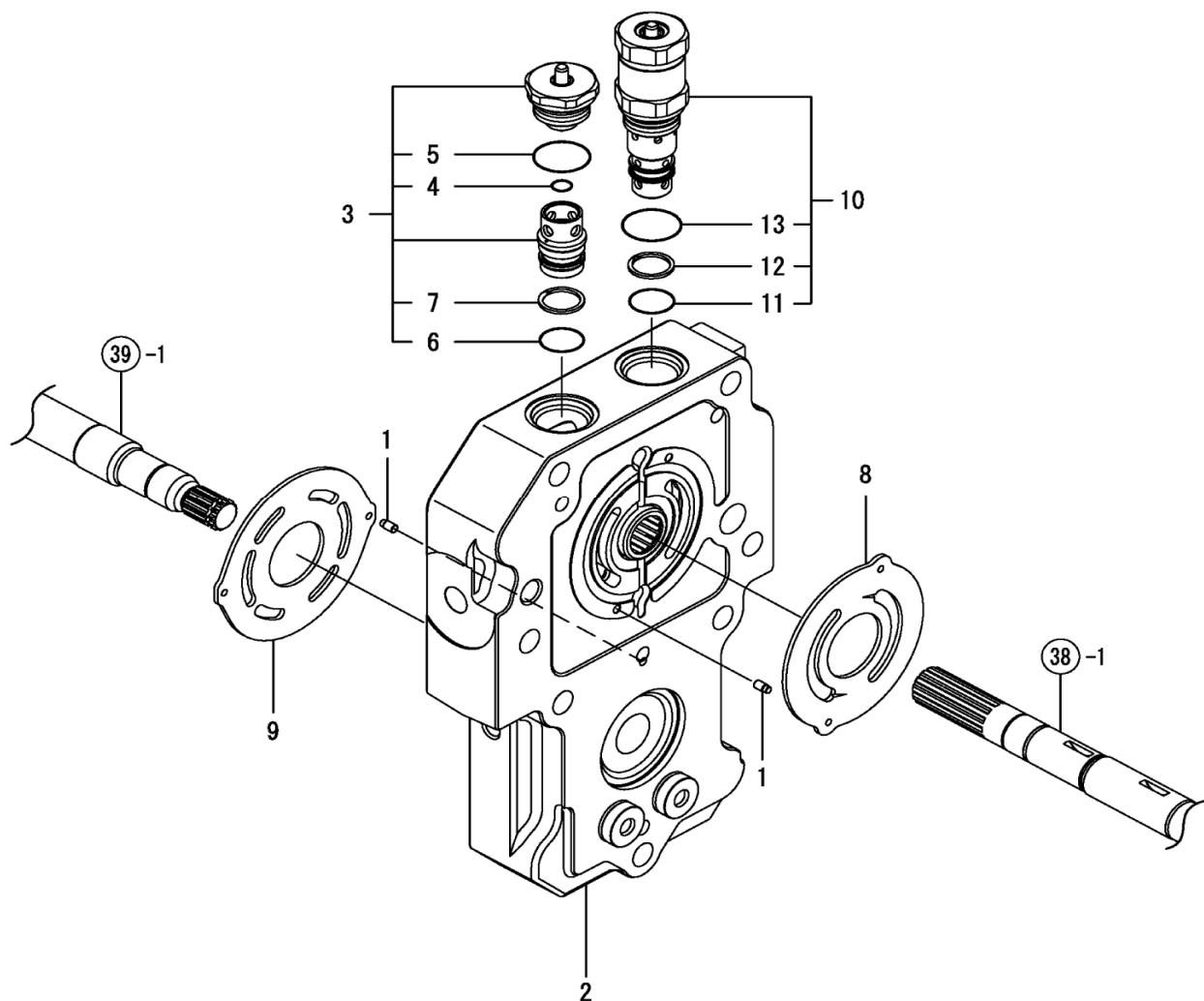
Fig. 35 - Center Case
