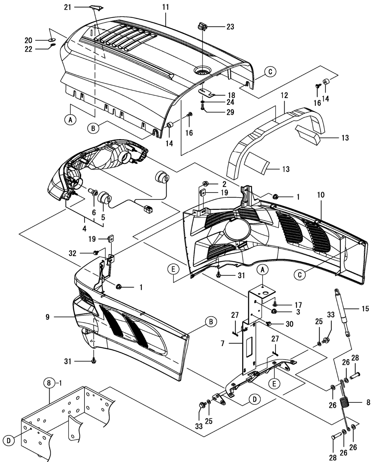
Fig. 87 - Hood
