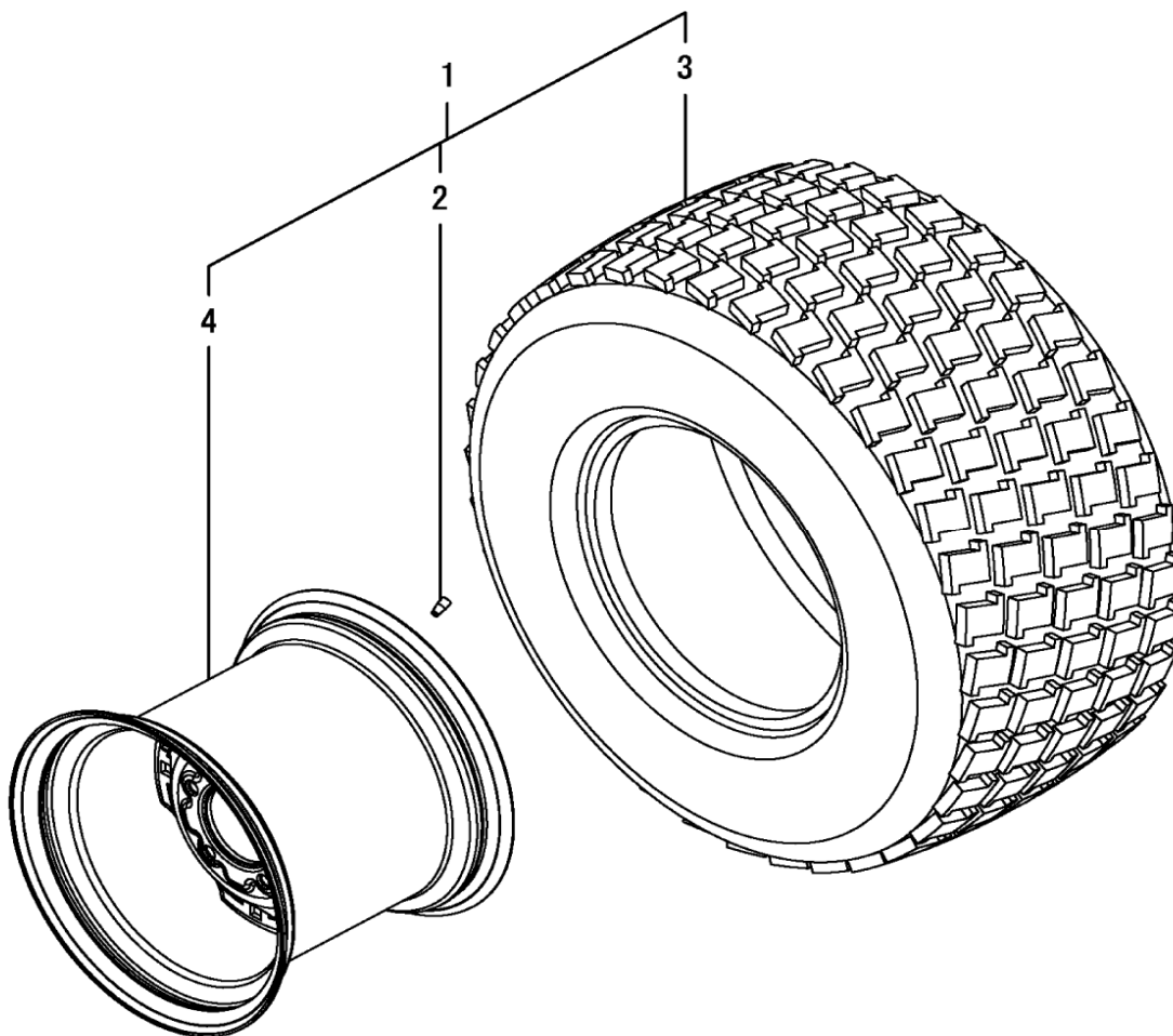
Fig. 64 - Tire, Rear (Turf)
