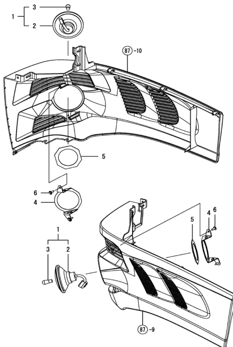
Fig. 85 - Side Lamp
