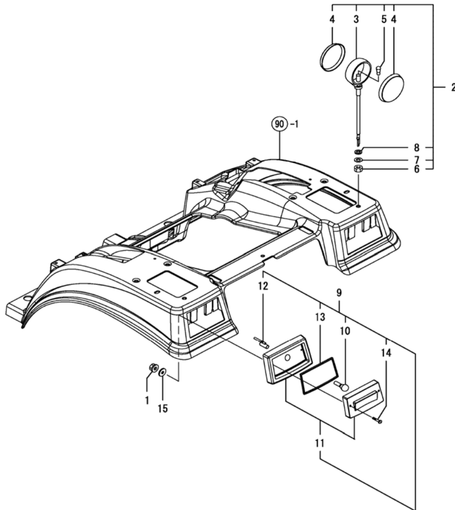
Fig. 84 - Lamps
