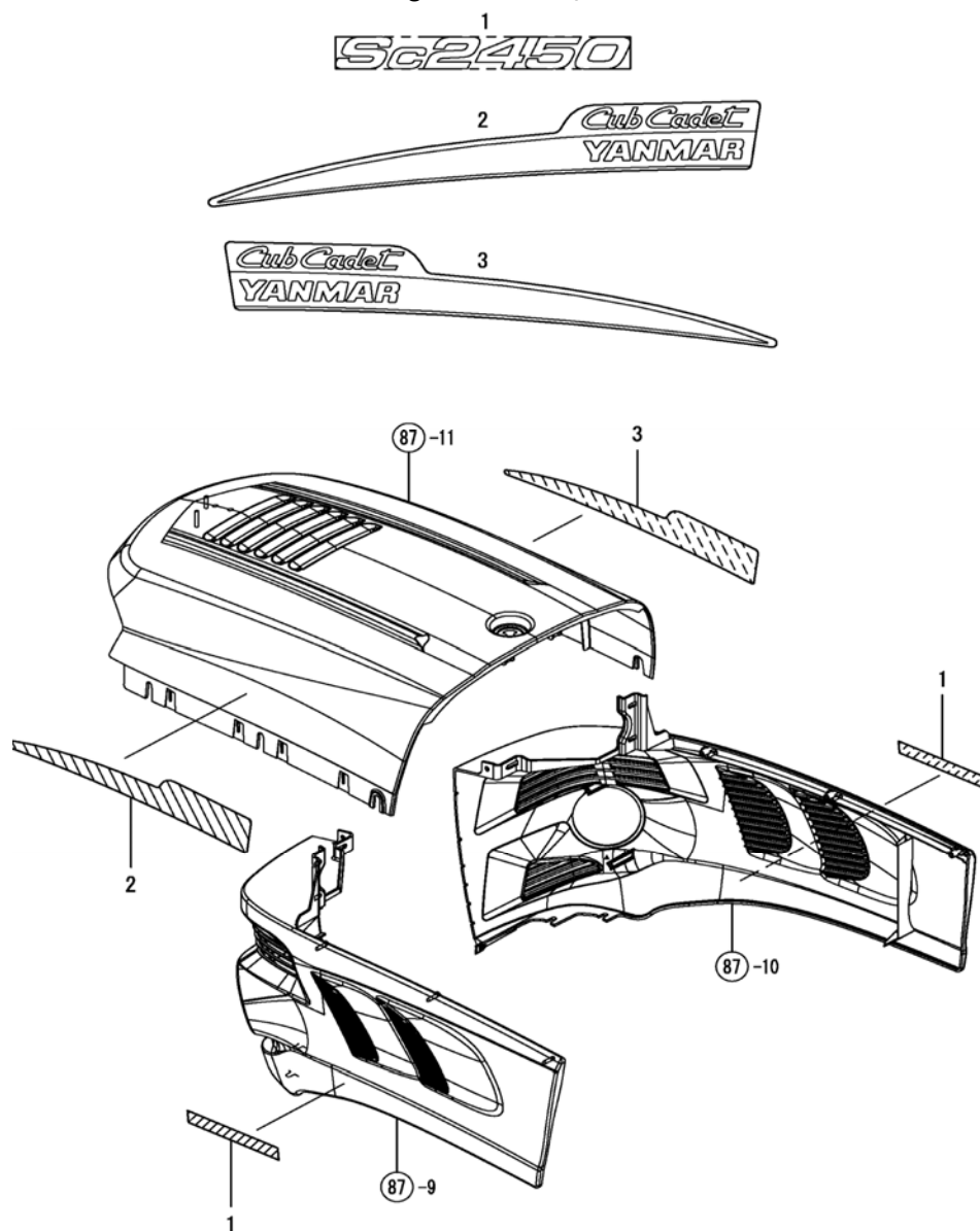
Fig. 97 - Label, Name
