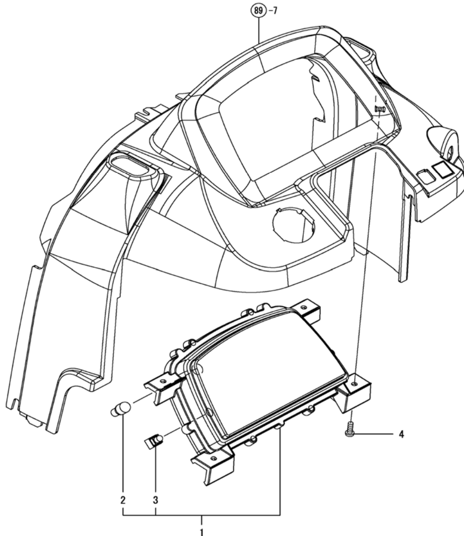
Fig. 86 - Meter
