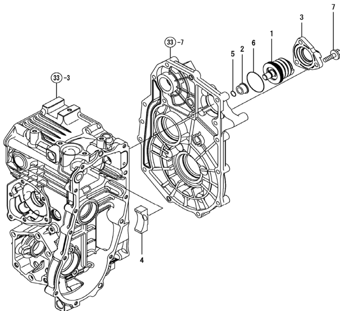
Fig. 41 - PTO Brake
