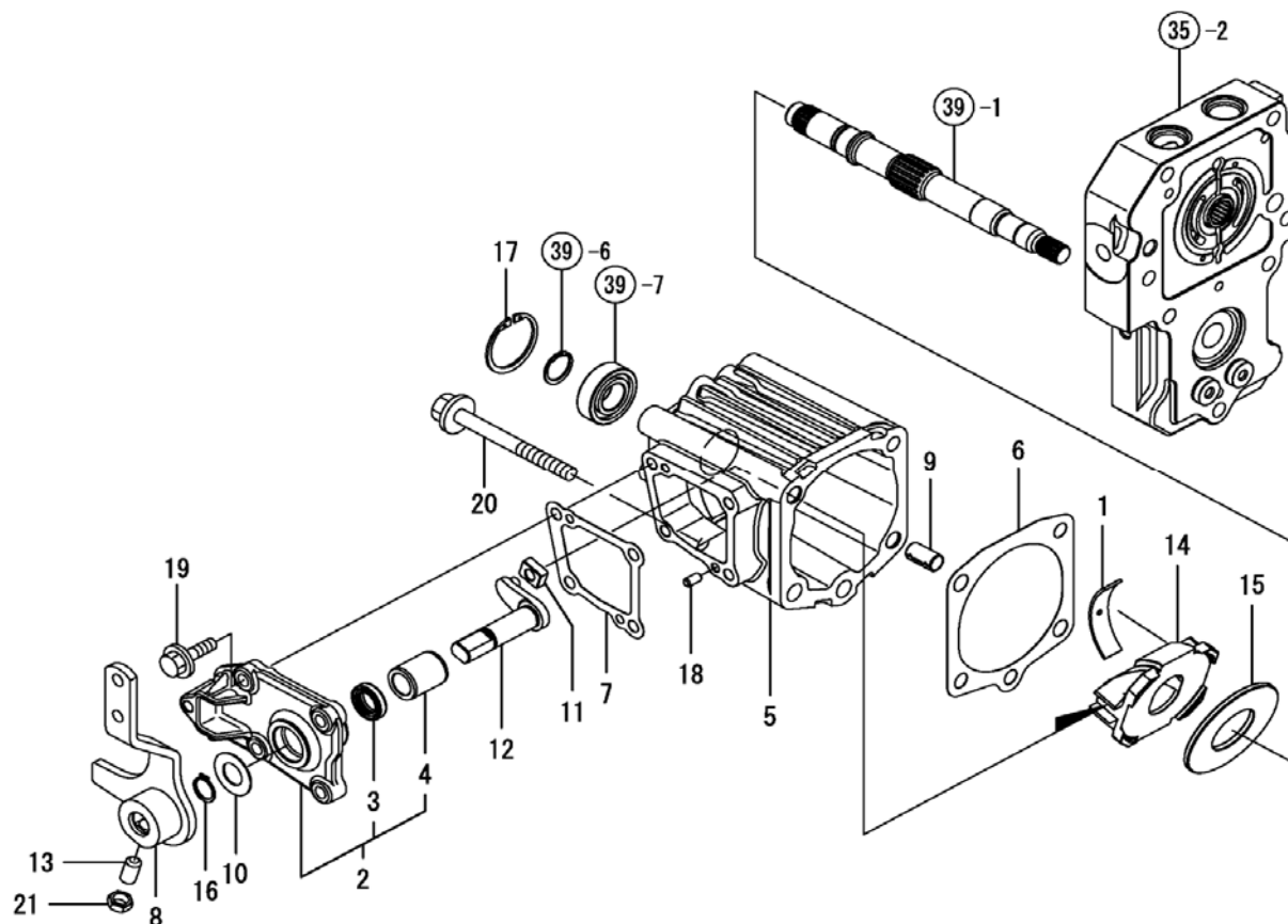
Fig. 36 - Motor Case
