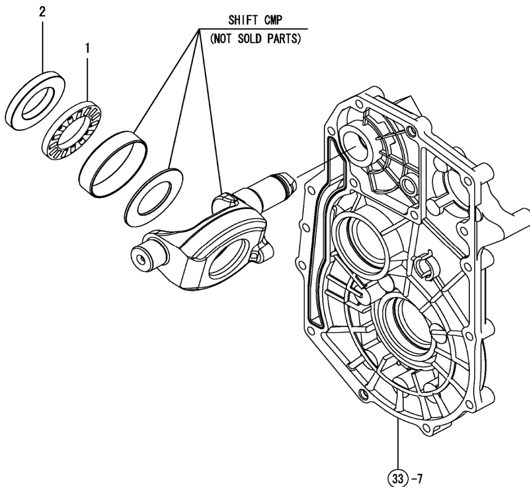
Fig. 46 - Shift
