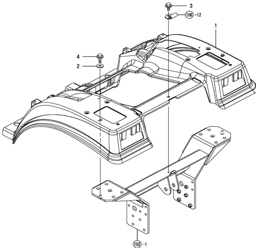
Fig. 90 - Fender
