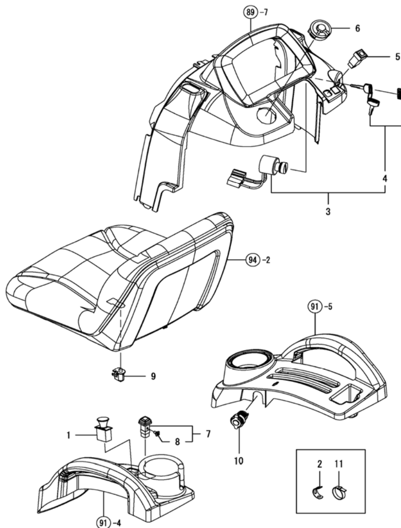
Fig. 83 - Switch B
