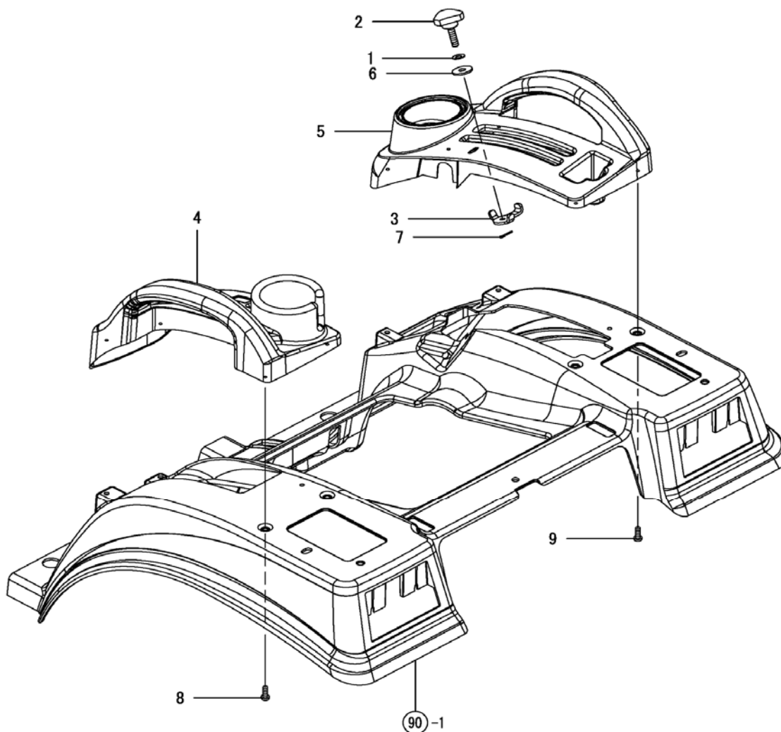
Fig. 91 - Lever Guide
