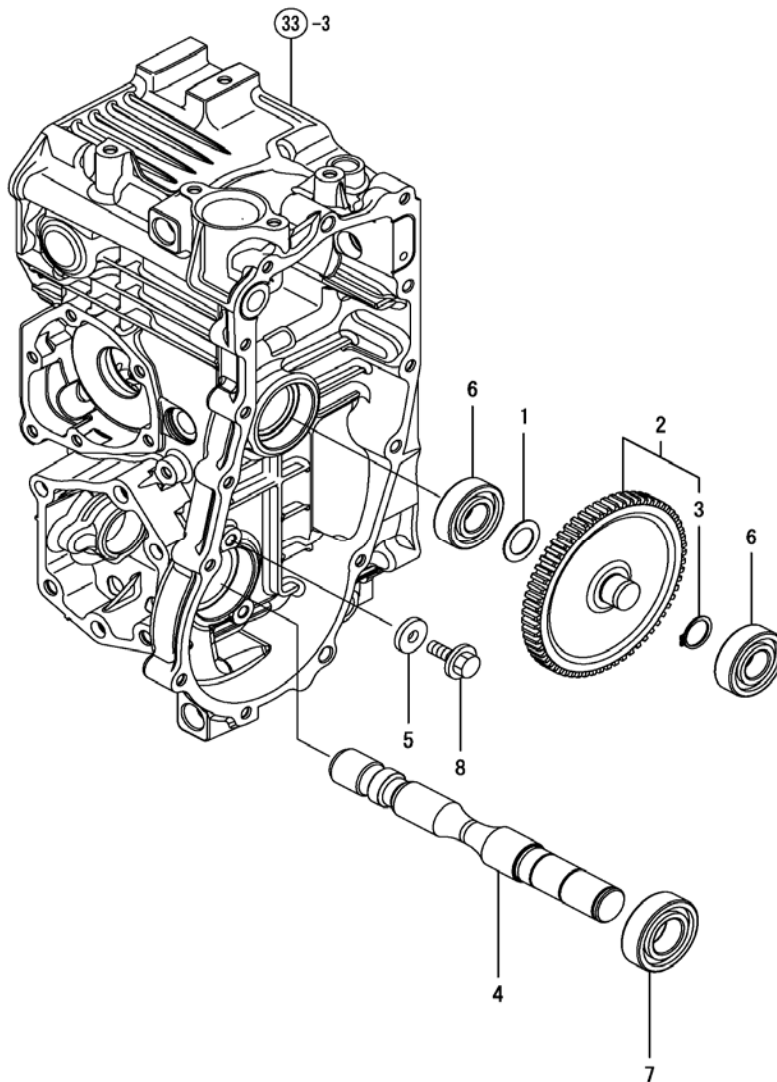
Fig. 42 - PTO Shaft
