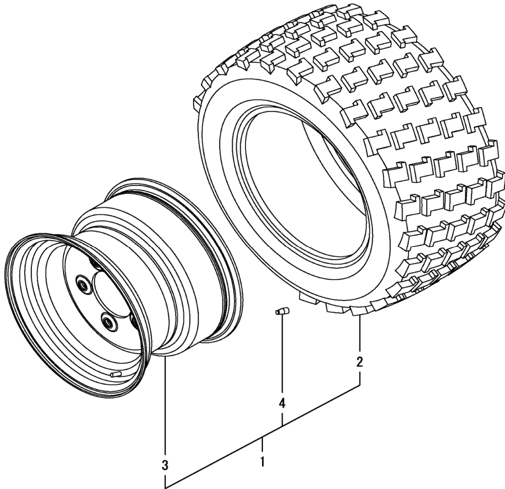
Fig. 23 - Tire, Front (Turf)
