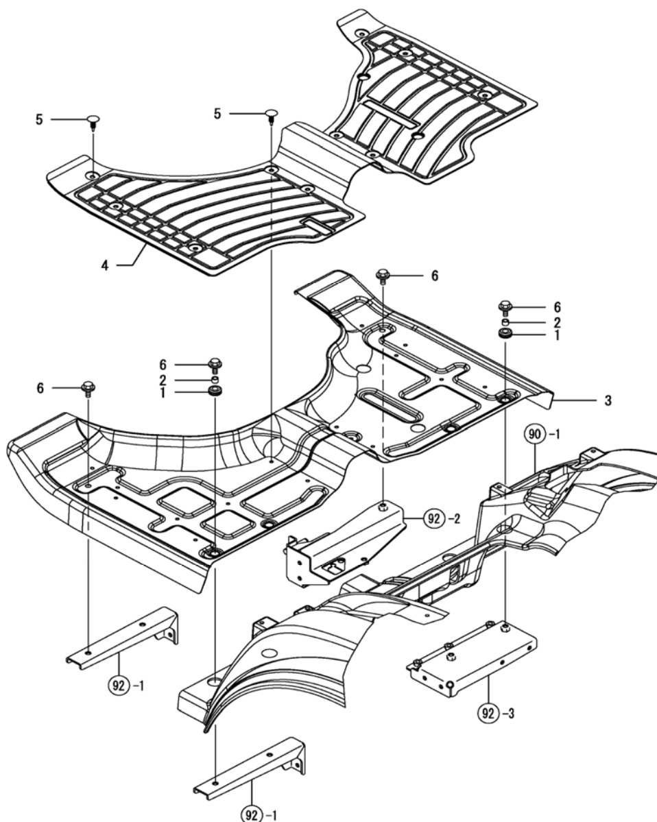
Fig. 93 - Step
