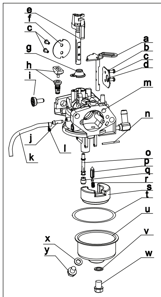
147 - Carburetor Rebuild Kit/ 147 - Trousse de reconstruction du carburateur
