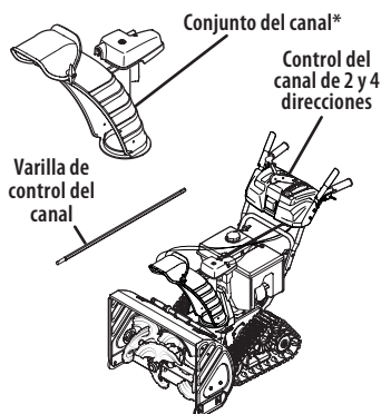
Control de Rotación del Canal Superior c/ Control de Rotación e Inclinación de 2 Direcciones o 4 Direcciones en la página 37
