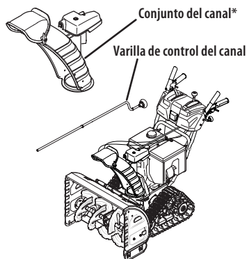
Control de Rotación del Canal Superior en la página 36
