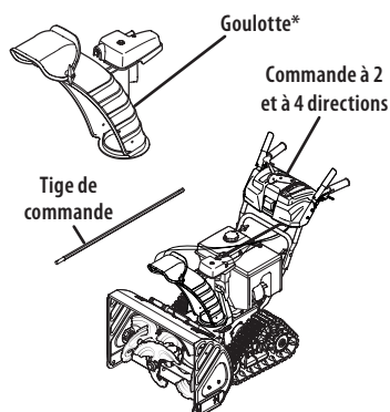
Commande supérieure de goulotte et commande de déflecteur à 2 ou à 4 directions à la page 66
