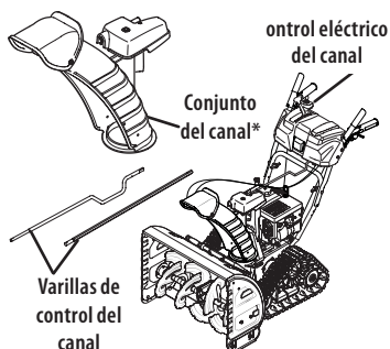
Control de Rotación del Canal Superior c/ Control Eléctrico de Rotación e Inclinación de 4 Direcciones en la página 40
