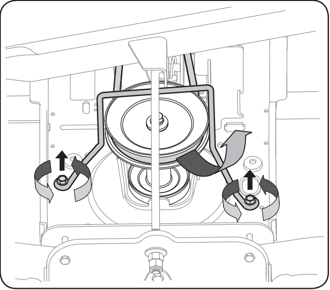
Figure 7-1 (Modèles avec prise de force manuelle illustrée) 4. Démontez le dispositif de protection de la courroie et la courroie comme suit. Voir la Fig. 7-1. a. Retirez la vis à six pans. b. Abaissez la tige du guide de la courroie vers la droite pour la retirer. c. Dégagez la courroie du plateau de coupe de la poulie motrice (ou de l'embrayage de la prise de force électrique, le cas échéant).
