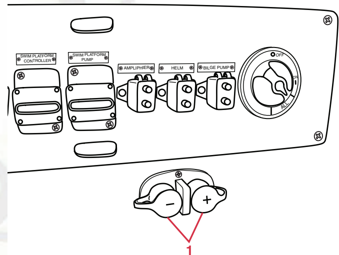
1 – Receptacle
