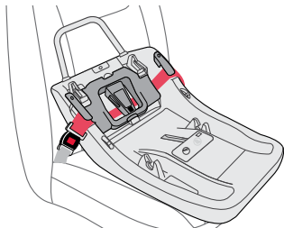
Instalación de la base con conectores inferiores
