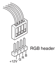
ARGB header
