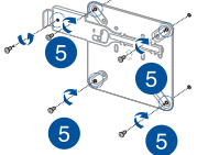
Tampilan bawah Mini PC
