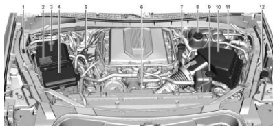
Moteur V8 6.2L suralimenté (LT4)
