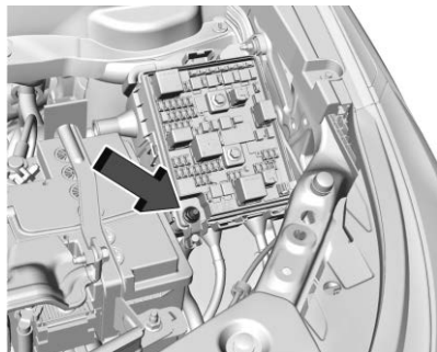
Terminal positiva (+) de batería descargada
